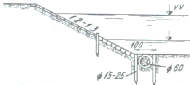
Obr. 8 Opevnění pomocí haťošterkových válců a dřevěných pilot [1]
