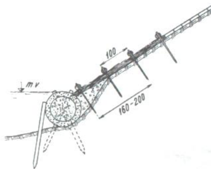
Obr. 5 Opevnění proutěným obkladem se zajištěním paty svahu pruto-šterkovým válcem [1]
