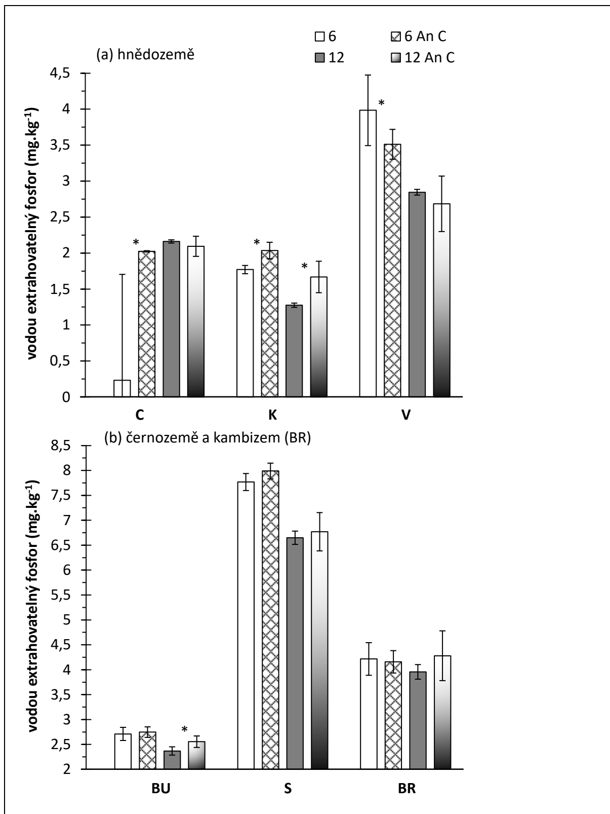
Graf 3(a),(b): Obsah vodou extrahovatelného fosforu ve vybraných půdních typech s odlišným ošetřením po 6 a 12 týdnech kultivace (zdroj: vlastní měření).
