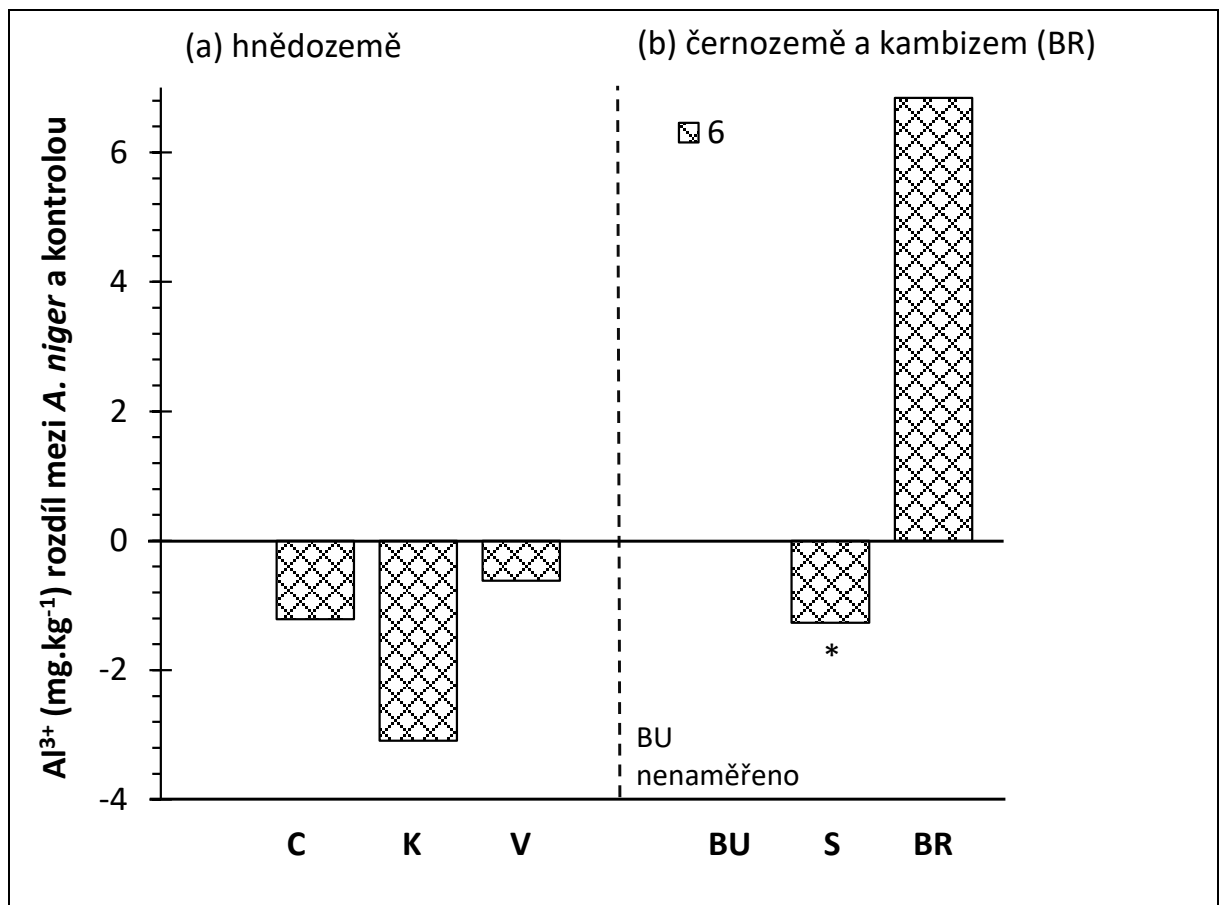
Graf 12(a),(b): Rozdíl v množství Al 3+ extrahovaný BaCl 2 mezi A. niger a kontrolou ve vybraných půdních typech po 6 týdnech kultivace (zdroj: vlastní měření).
