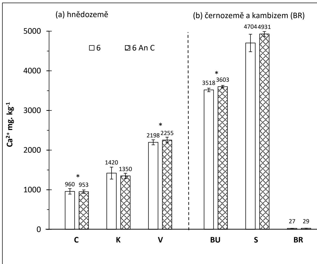
Graf 7(a),(b): Množství kationtu vápníku Ca 2+ stanoveného extrakcí BaCl 2 ve vybraných půdních typech s odlišným ošetřením po 6 týdnech kultivace (zdroj: vlastní měření).
