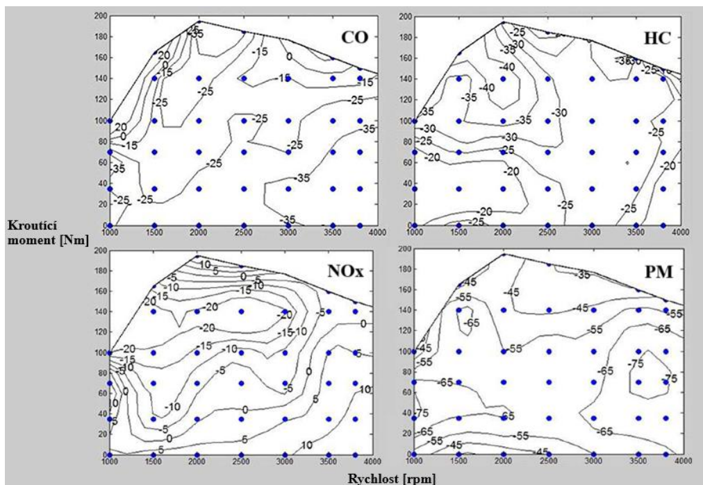
Obr. 7 Tvorba emisí při použití paliva HVO (upraveno) [21]
