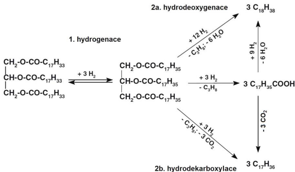
Obr. 4 Reakční schéma výroby HVO [19]
