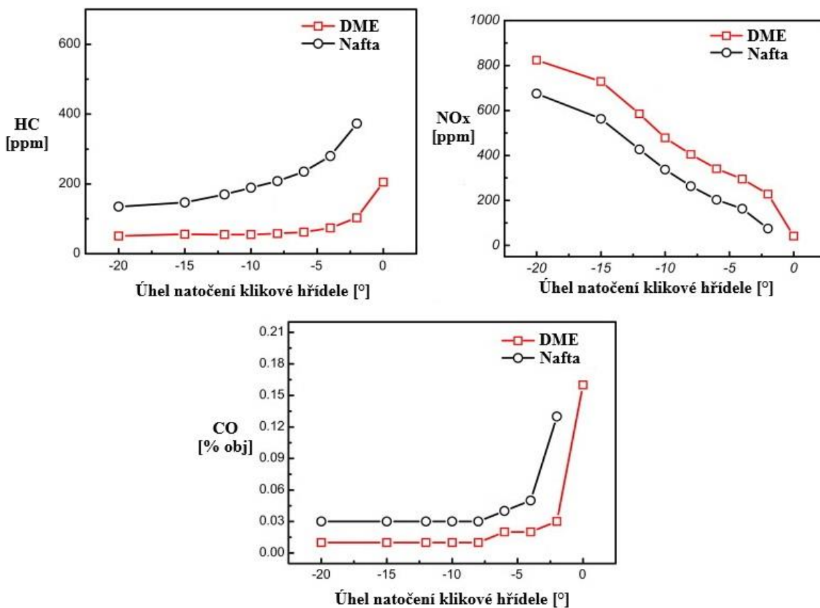
Obr. 10 Emise při spalování DME (upraveno) [26]
