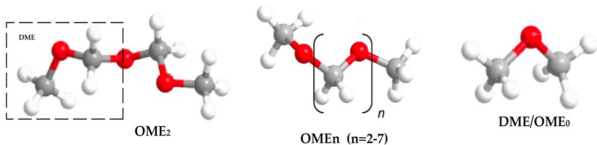
Obr. 9 Struktura paliv OME x a DME [24]
