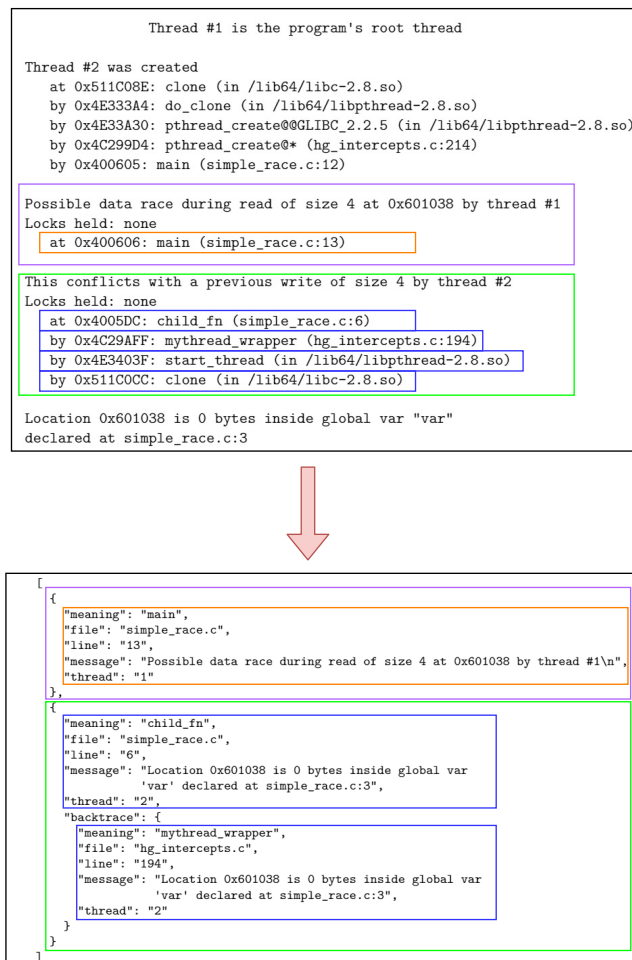
Obrázek 5.4: Ukázkový převod reportu do unifikovaného formátu.
