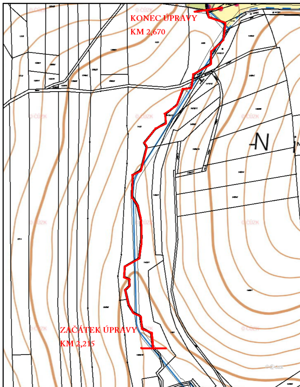
Obr. č. 33 Návrh směrového vedení toku (ČÚZK, © 2019)
