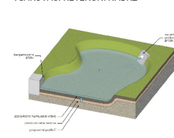
Obr. 75 - Vsakovací retenční nádrž, zdroj: 9
