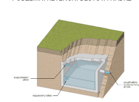
Obr. 76 - Podzemní retenční dešťová nádrž, zdroj: 9
