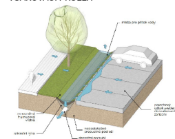
Obr. 73 - Vsakovací průleh, zdroj: 9
