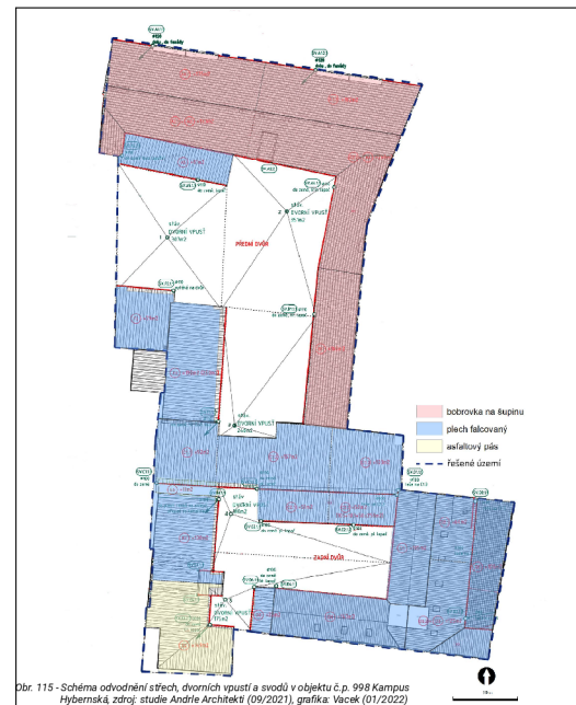
Dbr. 115 - Schéma odvodnění střešních, dvorních vpustí a svodů v objektu č.p. 998 Kampus Hyberská, zdroj: studie Andrie Architects (09/2021), grafika: Vacek (01/2022)
