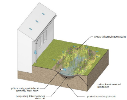
Obr. 72 - Dešťový záhon, zdroj: 9
