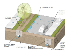
Obr. 74 - Vsakovací retenční rýha, zdroj: 9
