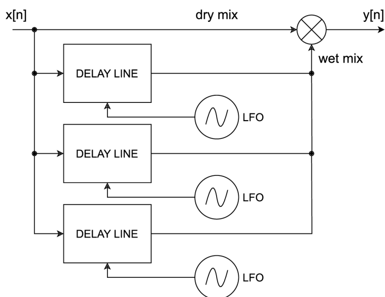
Obrázek 4.3: Schéma Chorus efektu.
