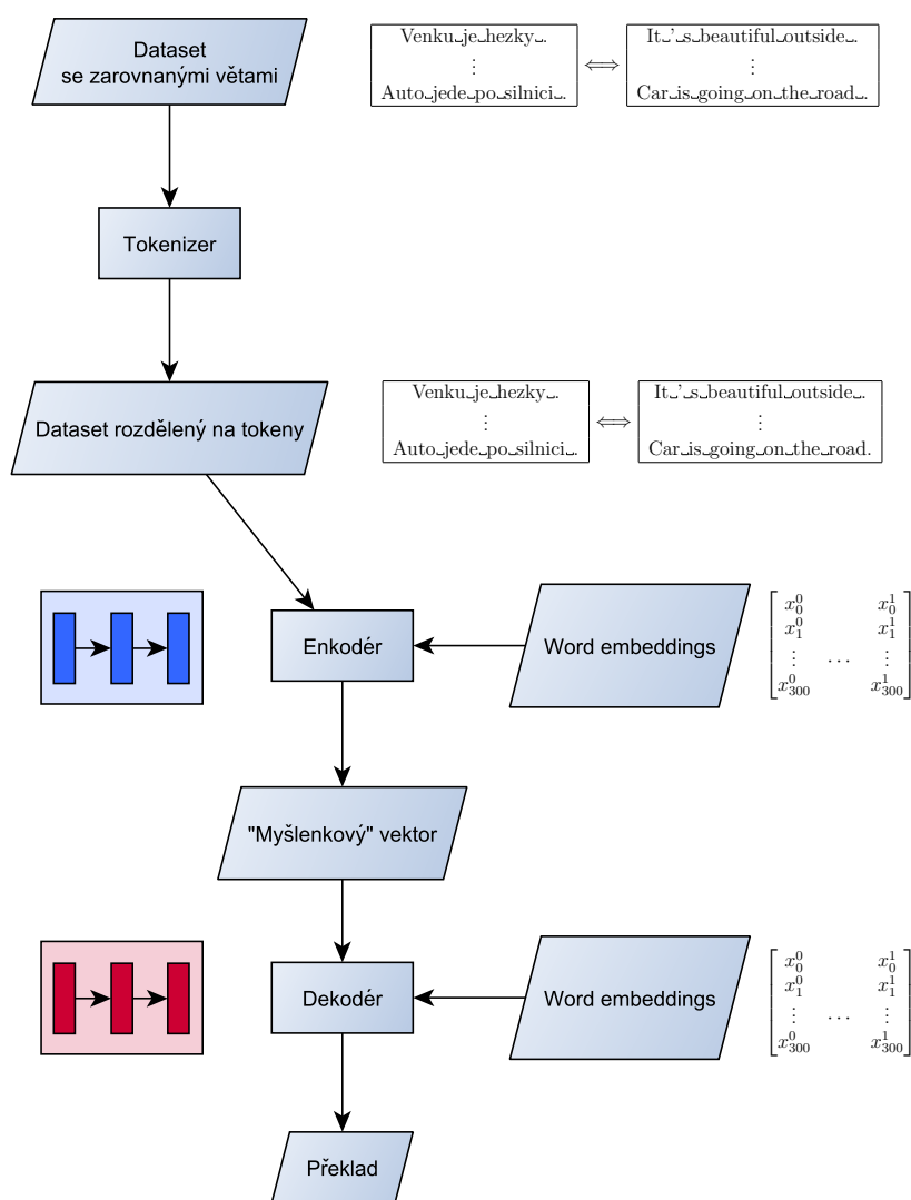
Obrázek 2.1: Schéma návrhu systému pro překlad. Dataset se předzpracuje pomocí tokenizera. Do enkodéru vstupují tokeny převedené na embeddings. Enkodér větu zakóduje do velkého "myšlenkového" vektoru, ze kterého dekodér generuje překlad.
