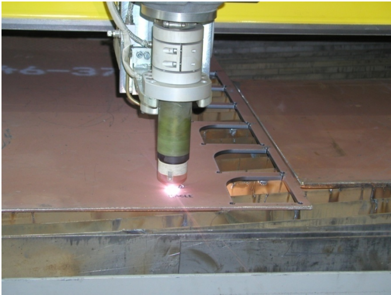
Obr. 6. 5 Řezání přesnou kyslíkovou plazmou[17]
