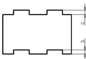
Obr. 2. 4 Minimální výška výstupků [11]
