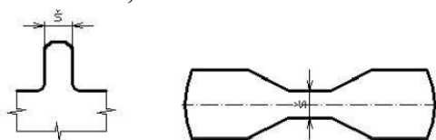
Obr. 2. 3 Minimální šířka výstřížku [11]
