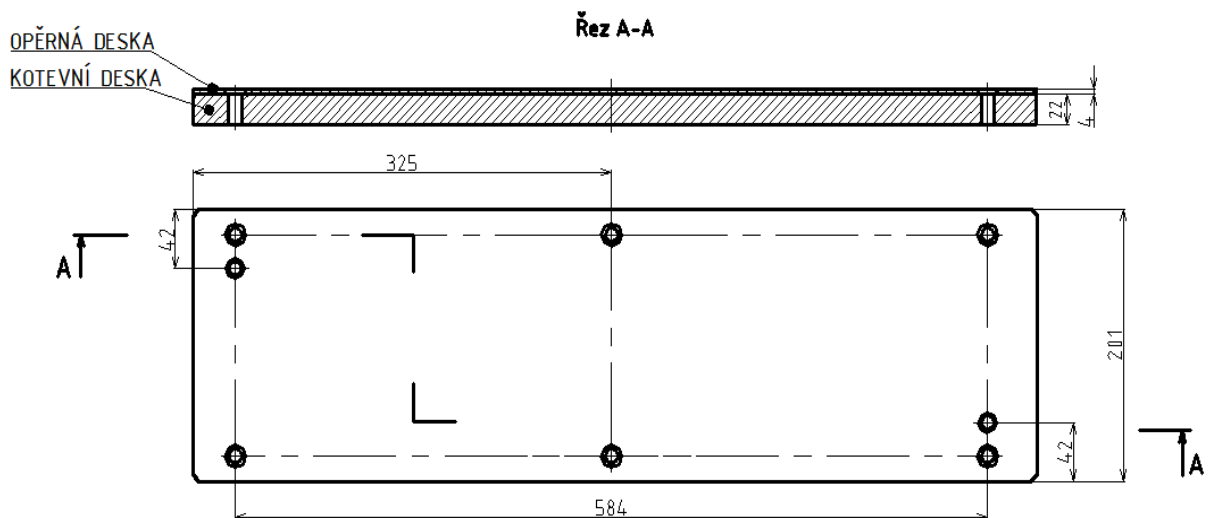
Obr. 3. 3. Hlavice 650 x 201
