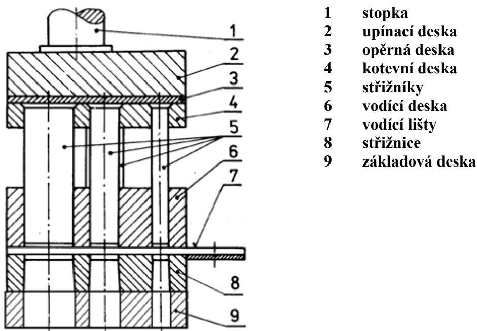
Obr. 3.1 Stříhací nástroj [11]
