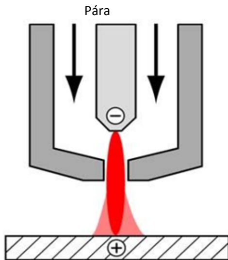
Obr. 6. 4 Přenášený (přímý) oblouk [15]
