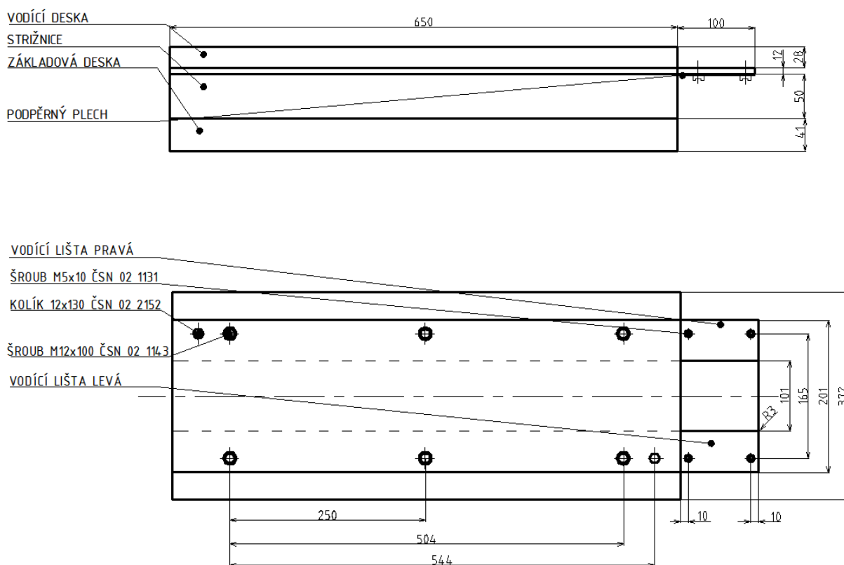
Obr. 3. 2. Střížná skříň 650 x 201
