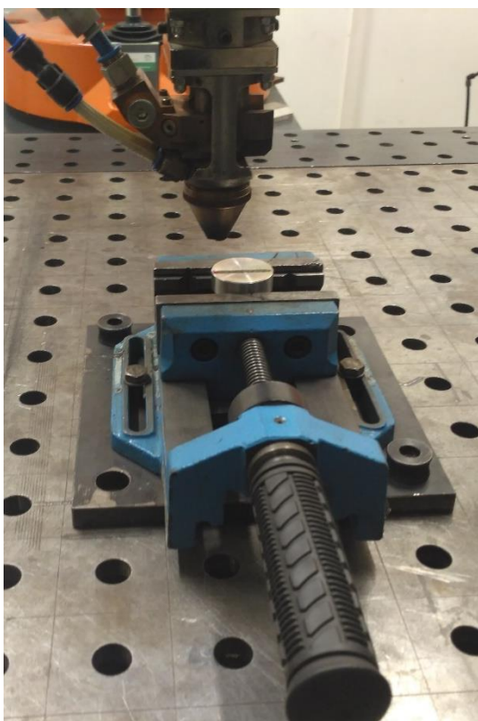
Obr. 26 Způsob upnutí vzorku.
