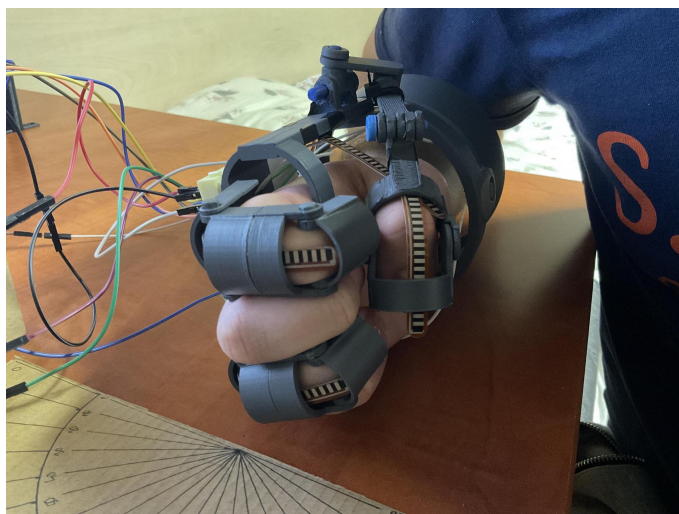
Obr. E.1: Vyvlieknutie senzorov pri meraní ohybu
