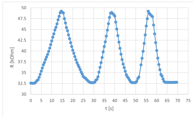
Obr. A.2: Závislosť senzoru 2 na rýchlosti ohybu
