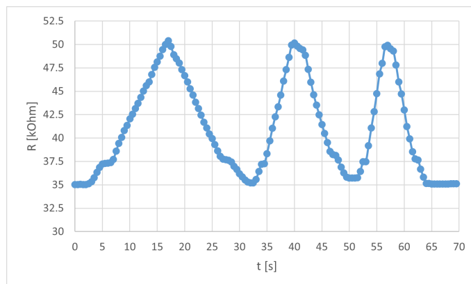
Obr. A.1: Závislosť senzoru 1 na rýchlosti ohybu
