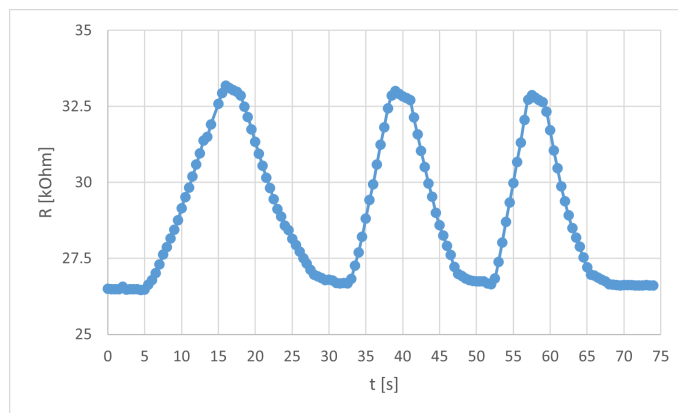
Obr. A.3: Závislosť senzoru 3 na rýchlosti ohybu
