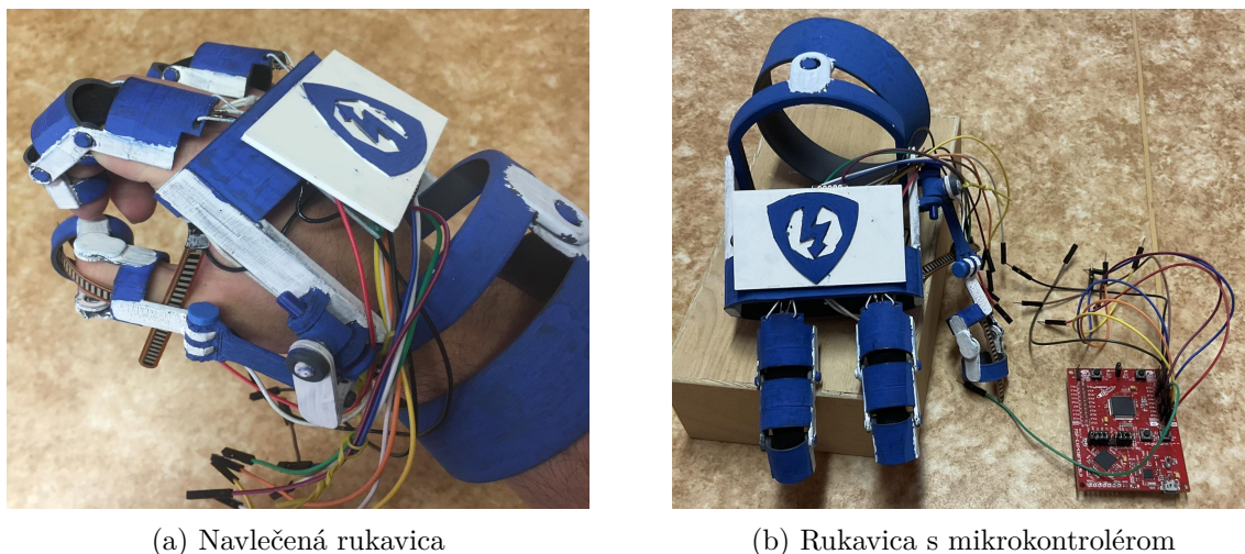
Obr. 10.1: Výsledná podoba dátovej rukavice
