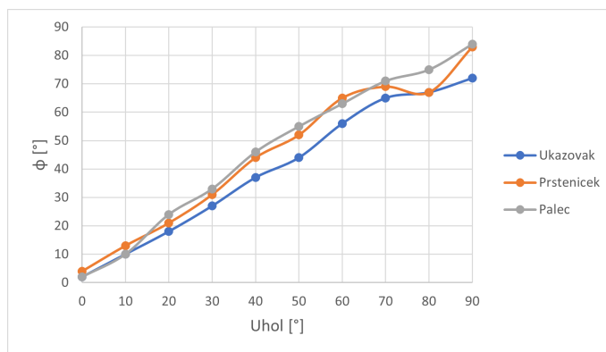
Obr. 8.2: Graf prvého merania ohybu prstov
