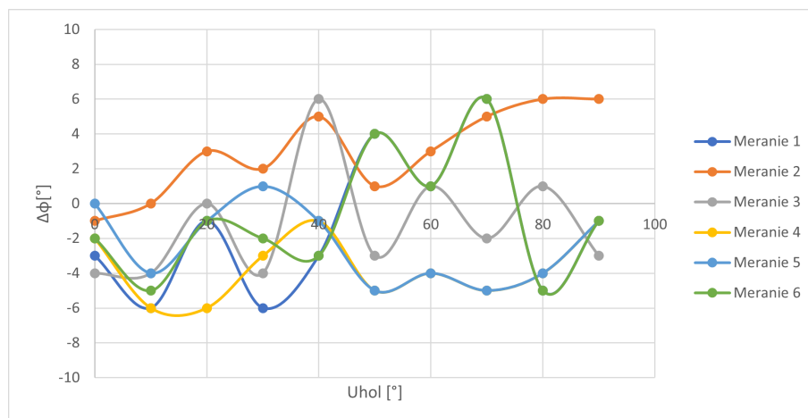
Obr. 8.5: Chyba merania pomocou výslednej rukavice - Ukazovák
