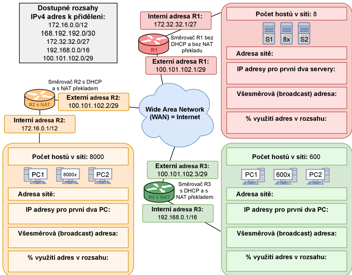
Obr. D.2.9: Šablona pro úkol č. (5) obsahující schéma sítí, pro které budeme hledat správný a co nejefektivnější rozsah při kombinaci veřejných a privátních adres.
