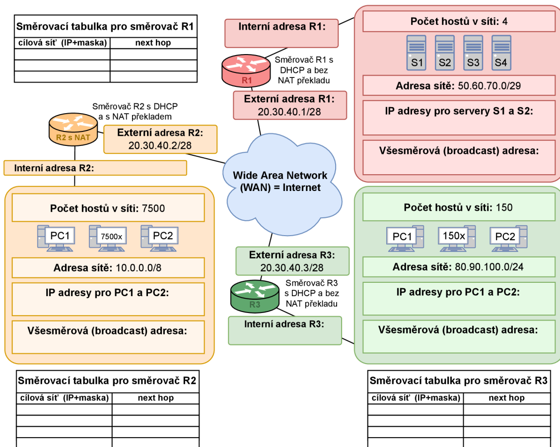
Obr. D.2.11: Šablona pro úkol č. (8) a (7) obsahující schéma sítí se směrovači R1, R2 a R3, pro které budeme doplňovat záznamy do jejich směrovacích tabulek.
