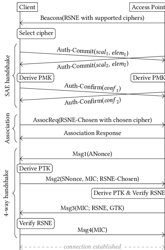
Obrázek 1: SAE Handshake [31]
