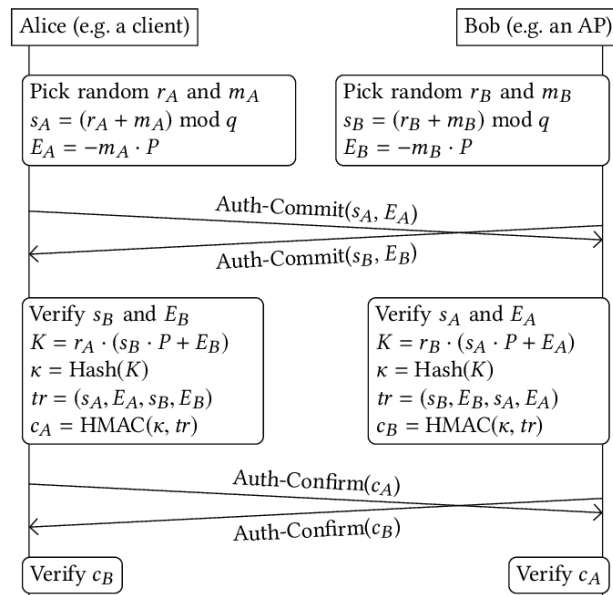
Obrázek 2: SAE Handshake2 [31]
