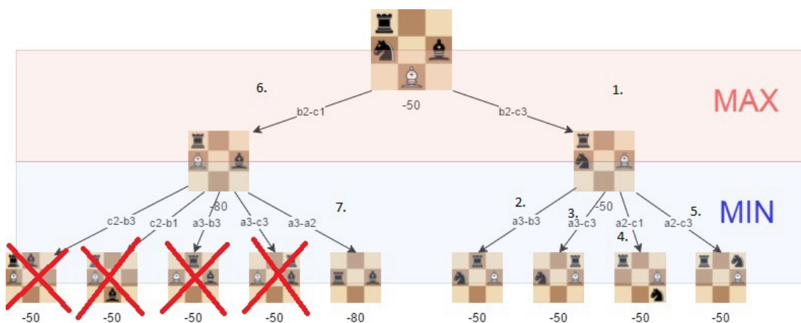
Obr. 8 Ukázka algoritmu Alfa-beta ořezávání Zdroj: (11)
