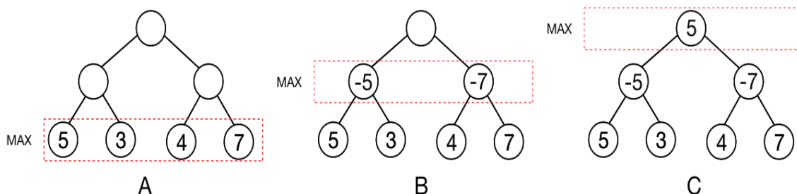
Obr. 9 Algoritmus NegaMax
