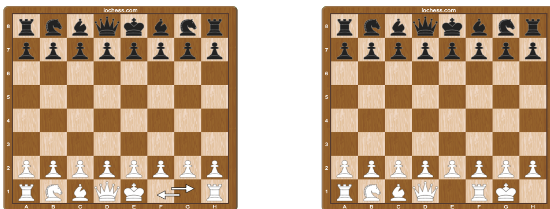
Obr. 3 Rošáda „kingside“
