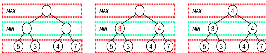
Obr. 4 Algoritmus MinMax
