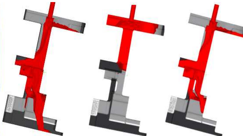
Obr. 2.4-65 15s: Skut., sim. č.5, sim. č.3, sim. č.1
