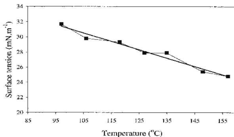
Graf 2.4-3 Povrchové napětí v závislosti na teplotě [26]
