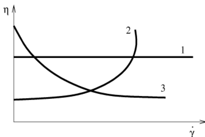
Obr. 1.5-8 Viskózní křivky pro kapaliny : 1) newtonovská , 2) dilatantní newew., 3) pseudoplastická newew.
