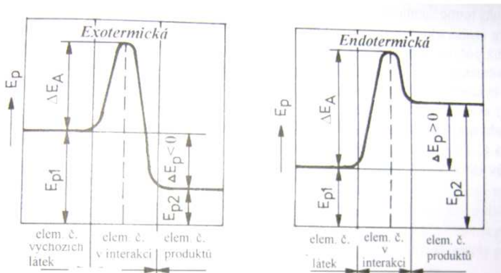
Obr. 1.5-5 Změny potencionální energie elementárních částic v průběhu reakce [37]
