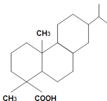
Obr.1.6-5 Příklad řetězce hydrogenované pryskyřice [10]
