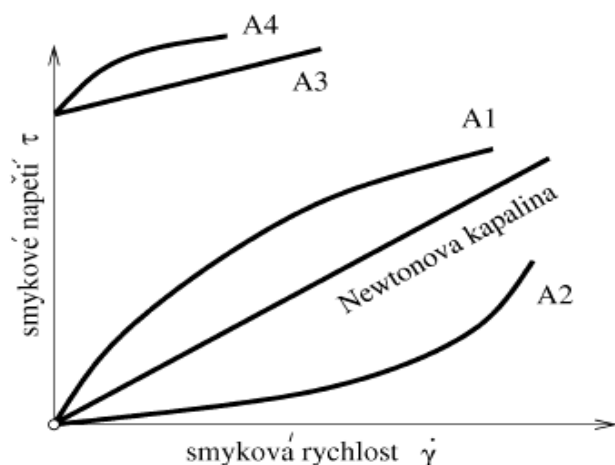
Obr. 1.5-7 Tokové křivky (reogramy) pro obecně viskózních newew. kapalin A1 – pseudoplastická, A2 – dilatantní, A3 – Binghamova, A4 – Cassonova
