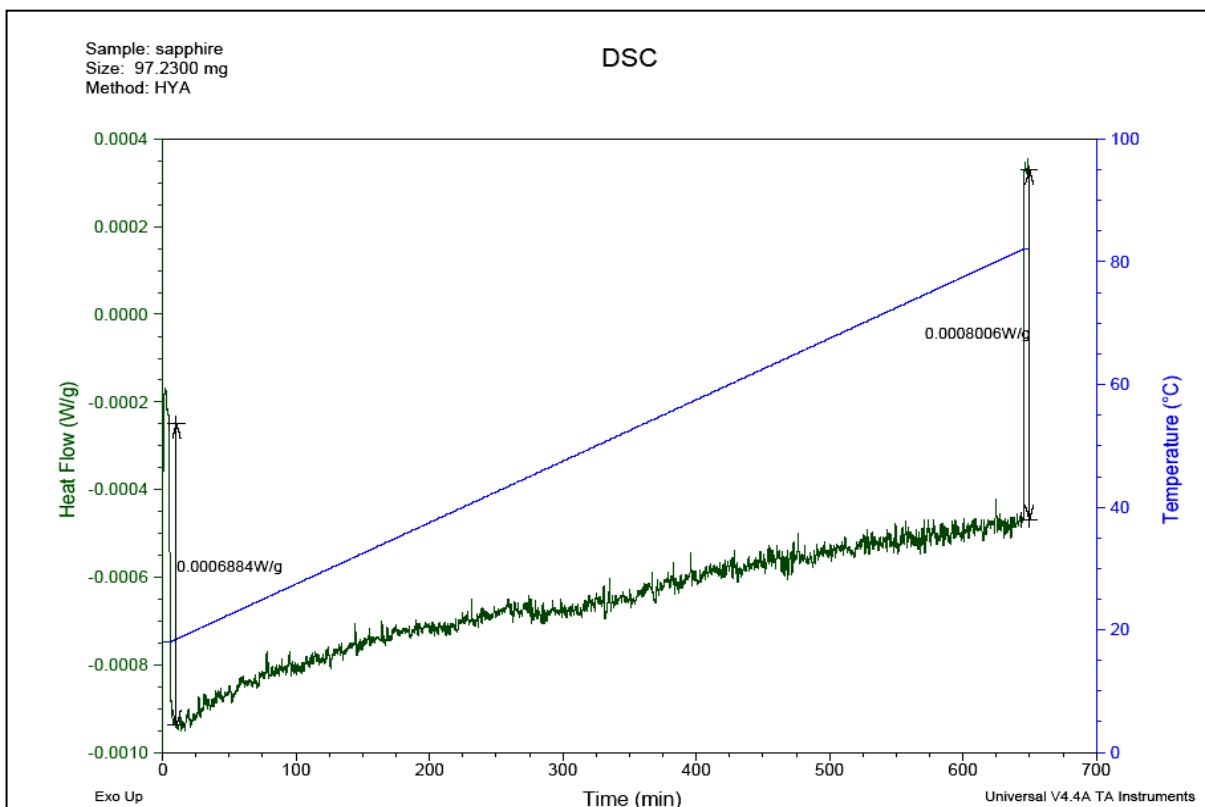
Graf 2.4-15 Závislost tepelného toku na čase a teplotě pro porovnávací vzorek – safir
