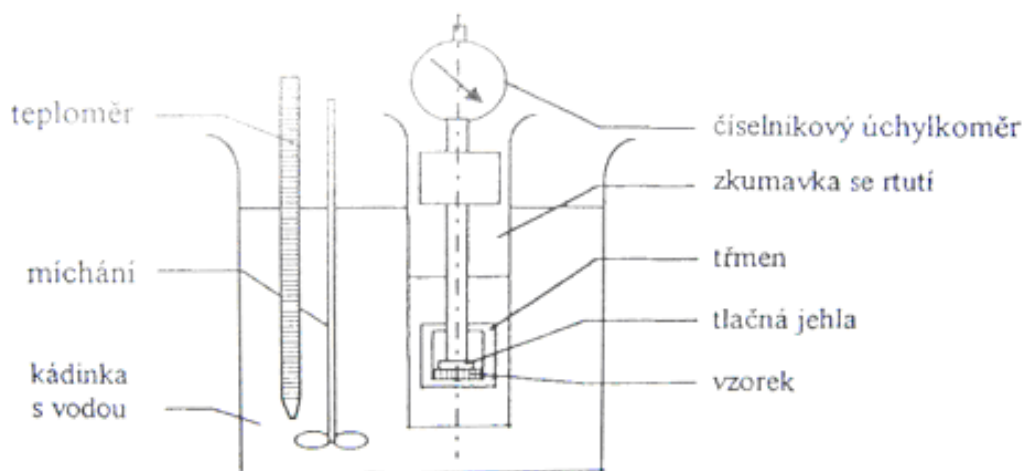
Obr.1.6-10 Určení bodu tání penetrometricky [41]
