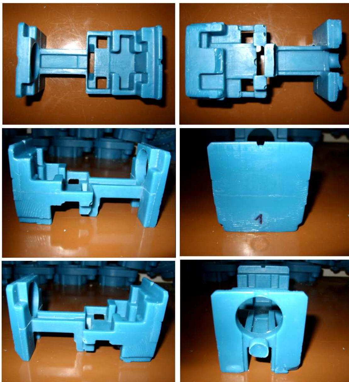
Obr. 2.2-16 První odlitý voskový odlitek, úhel sklonu formy 20°, čas lití cca 120 s, vakuum při lití -0,6 Bar, lící teplota voskové směsi 70 °C, teplota předehřátí formy 70 °C. Forma neprodyšná – bez průduchů.
