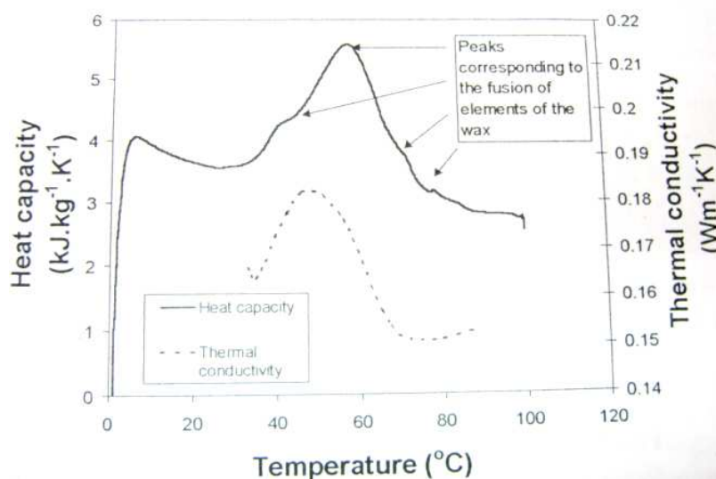
Graf.1.5-1 Známořuje průběh křivek tepelné kapacity a tepelné vodivosti v závislosti na teplotě [26]
