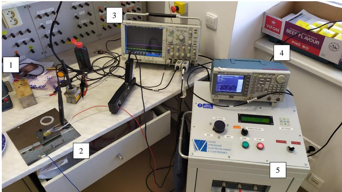
Obrázek 21 – Měřicí pracoviště
