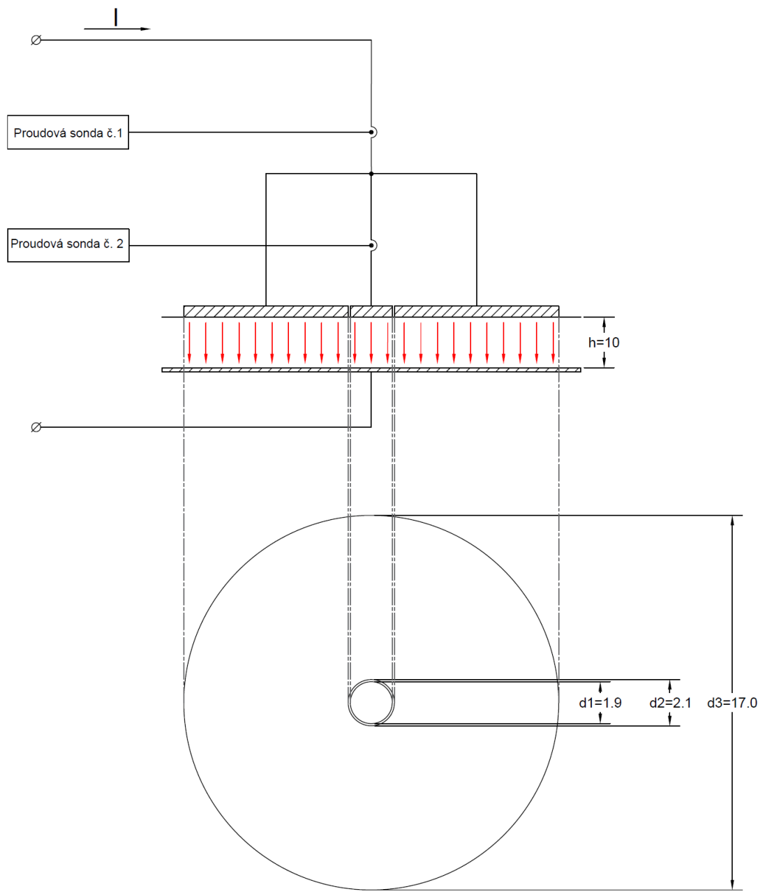
Obrázek 22 – Detailní náčrtek měřícího přípravku
