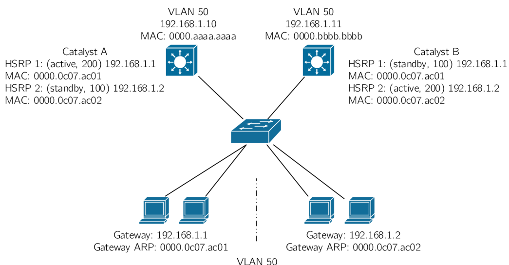
Obrázek 2.2: Příklad load balancingu při použití dvou HSRP skupin. Převzato z [11].
