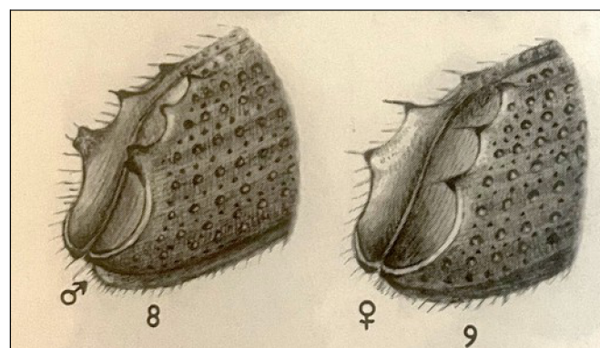
Obr. č. 4 - Dimorfismus u Ips acuminatus (Pfeffer, 1989)
