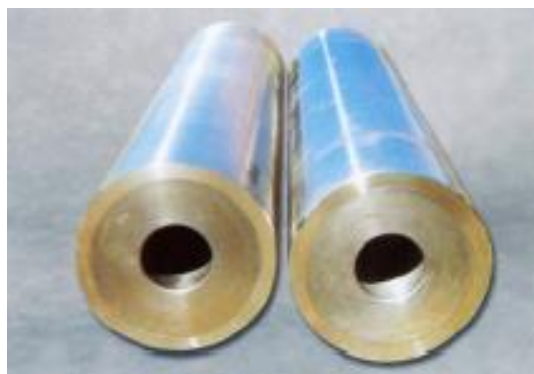
Obr.44: Dvouvrstvé mlecí válce (vnější vrstva z tvrdé, vnitřní vrstva z šedé litiny) [20]
