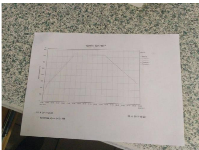
Obr.33: Graf tepelného zpracování (teplota na čase)
