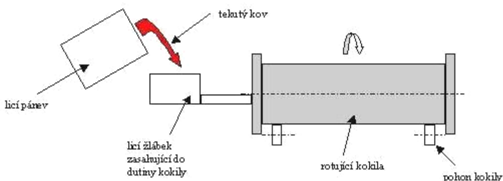
Obr.3: Princip odstředivého lití do kovové formy [24]
