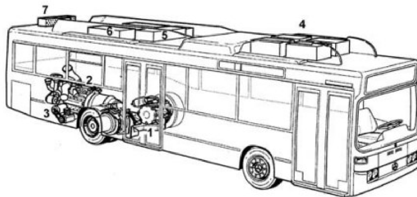
1 – motor v náboji kola; 2 – vznětový motor s generátorem; 3 – vzduchový kompresor a čerpadlo servořízení; 4 – trakční baterie; 5 měnič palubní sítě; 6 – měnič elektrické-ho proudu; 7 – brzdový odpor.
