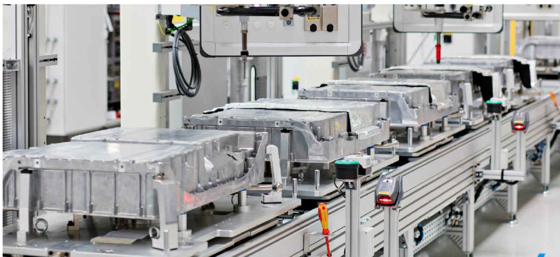
Obr. 2.9 Montážní linka pro baterie technologie PHEV
