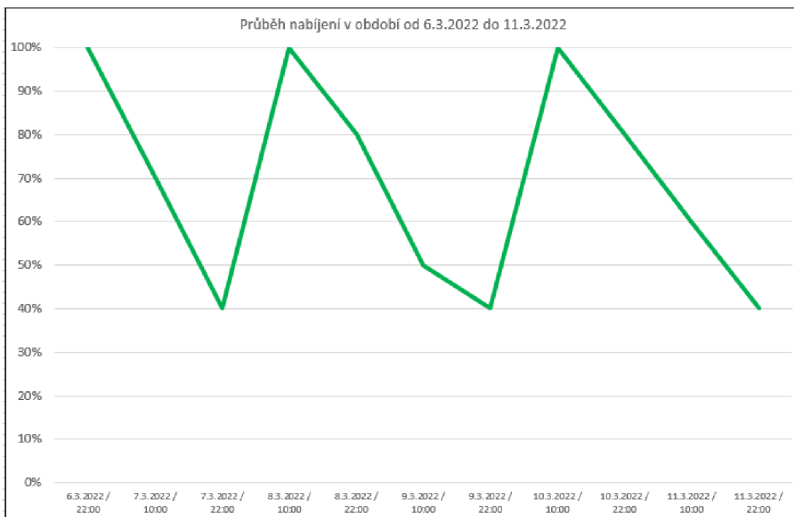
Graf 3.1 Grafické znázornění průběhu nabíjení v KT10
