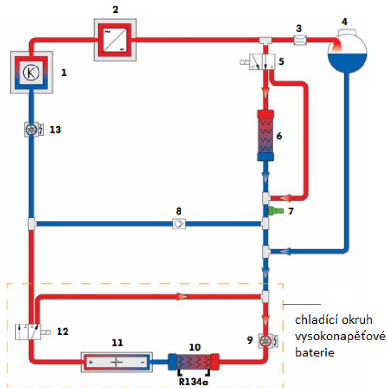
Schéma 2.1 Chladicí okruh pro vysokonapěťové komponenty
