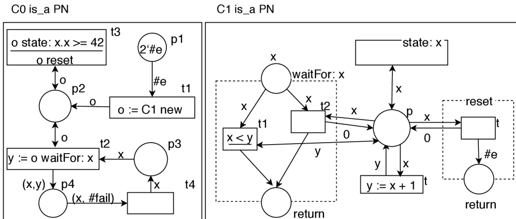
Obrázek 2.2: Grafický zápis OOPN.
