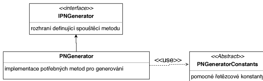
Obrázek 4.6: Model tříd generátoru.
