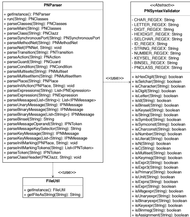
Obrázek B.2: Model tříd syntaktického analyzátoru.
