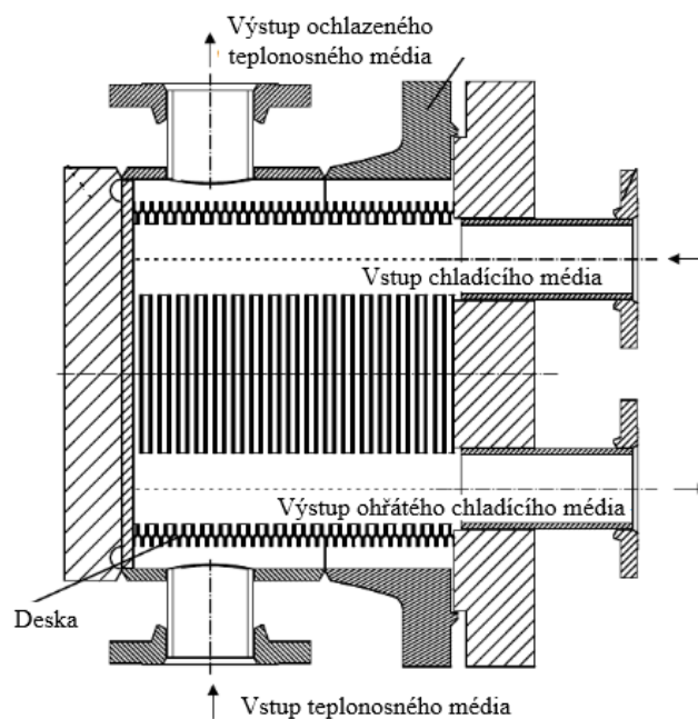
Obr. 21 Schematické zobrazení plášťovo deskového výměníku [24] (upraveno).
