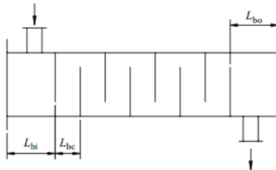
Obr. 27 Schematické zobrazení roztečí přepážek [32].
