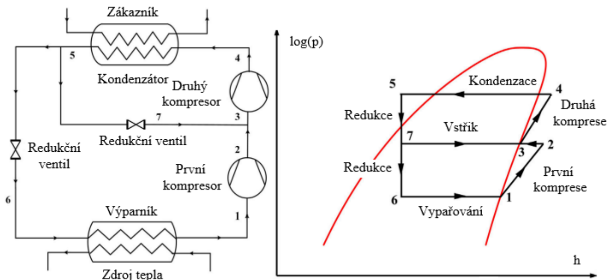
Obr. 7 Dvoustupňové tepelné čerpadlo s vnitřním vstříkem a p-h diagram [7] (upraveno).
