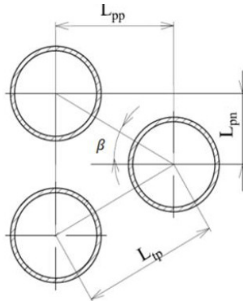
Obr. 25 Schematické zobrazení uspořádání a roztečí trubek [31].
