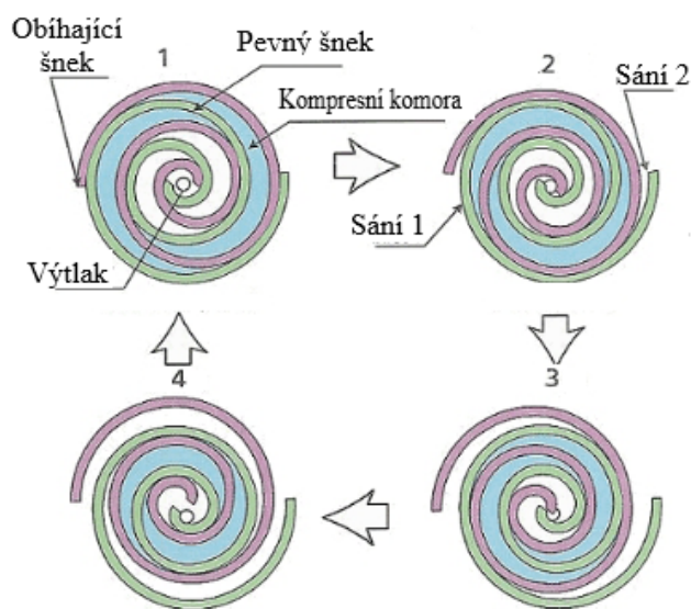
Obr. 14 Cyklus stlačování spirálového kompresoru [16] (upraveno).
