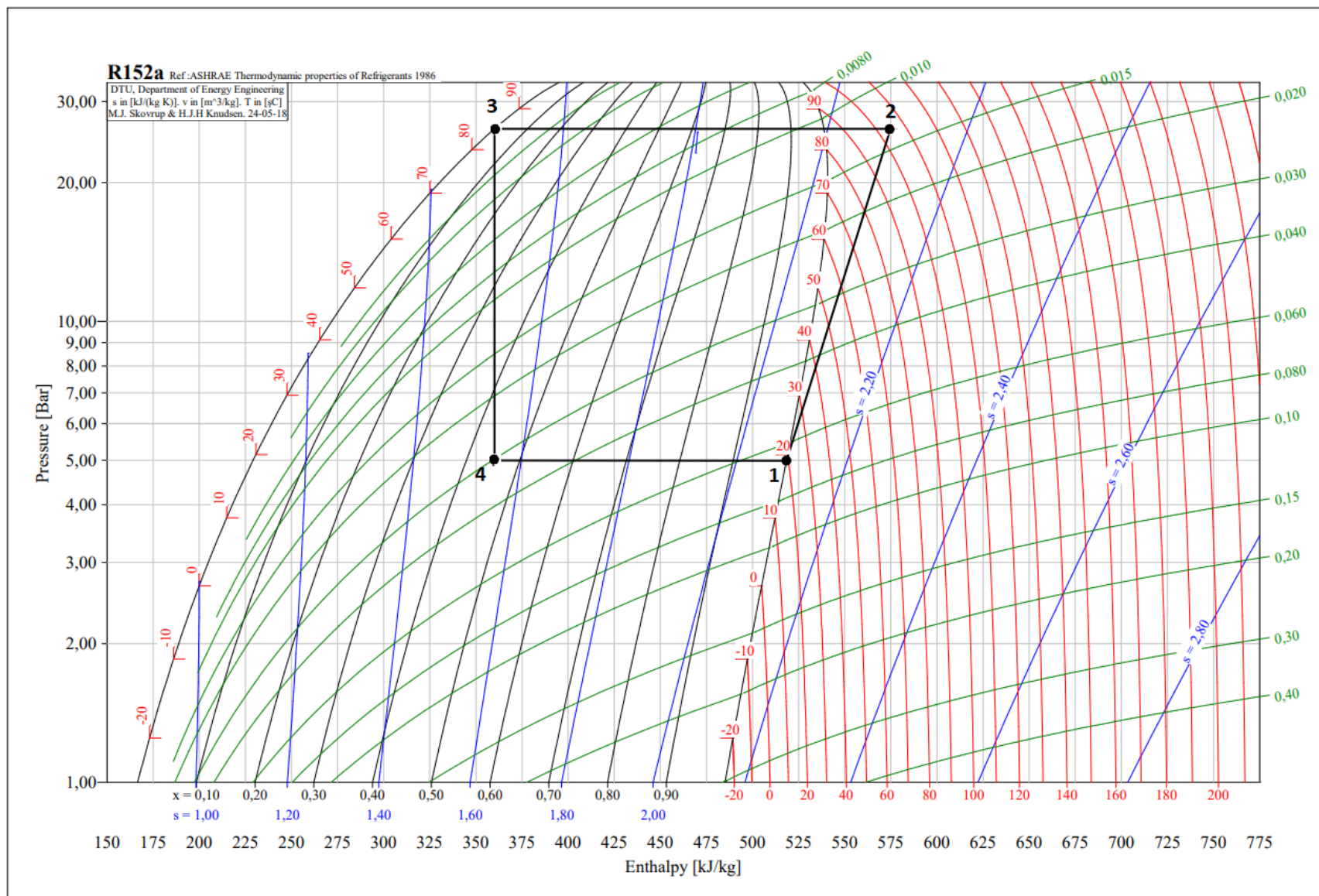
Obr. 33 P-h diagram reálného pracovního cyklu tepelného čerpadla [29].
