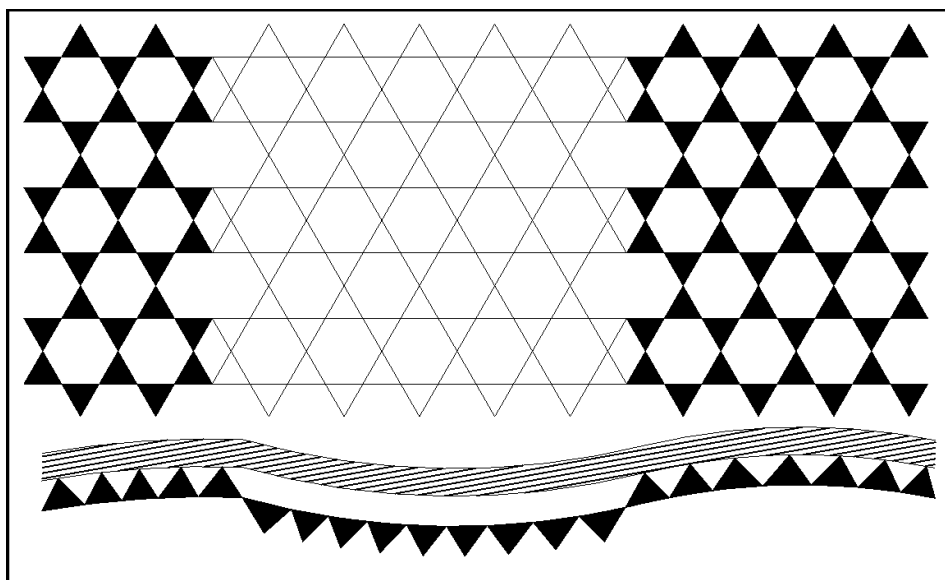
Obrázek 8: Schematické zobrazení modulované struktury 1:1 fylosilikátu. Modulovaná je tetraedrická síť jež vytváří pásy tetraedrů s opačnou polaritou a oktaedrická síť zůstává kontinuální (naznačeno šrafováním). Nahoře je strukturní model v pohledu kolmém na vrstvy a dole rovnoběžně s vrstvami. [11]
