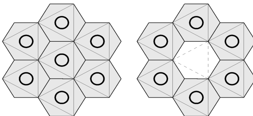
Obrázek 5: Výsek idealizované trioktaedrické sítě (vlevo) a dioktaedrické sítě (vpravo) v pohledu kolmém na rovinu aniontů. Oktaedrické pozice jsou označeny kroužkem.
