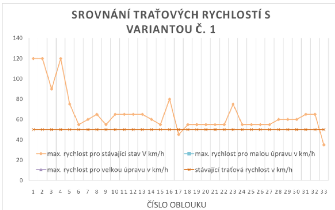
Obr.3.1-2 Srovnání rychlostí
