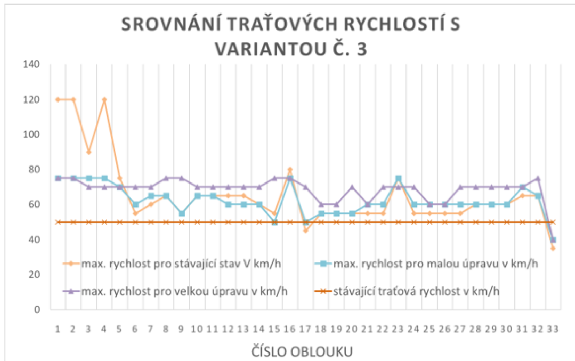
Obr.3.3-4 Srovnání rychlostí 3
