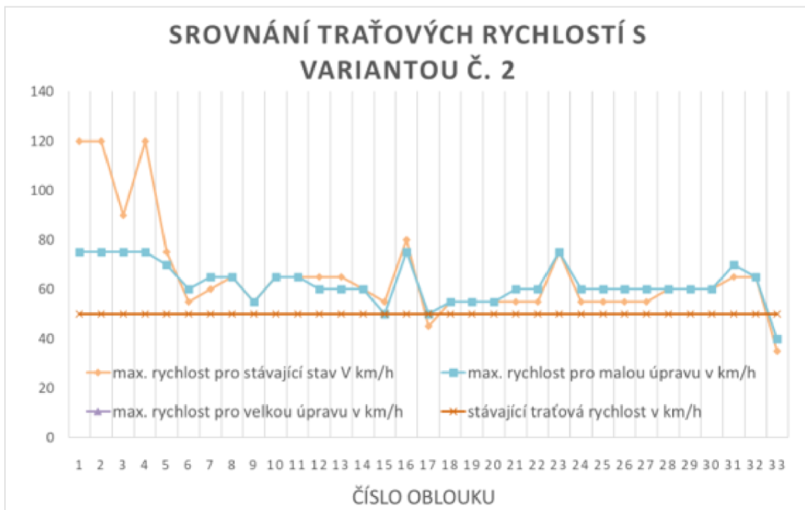
Obr.3.2-3 Srovnání rychlostí 2
