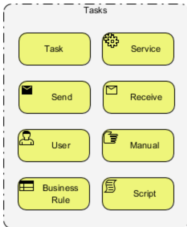
Obr. 15 Základní druhy BPMN aktivit
