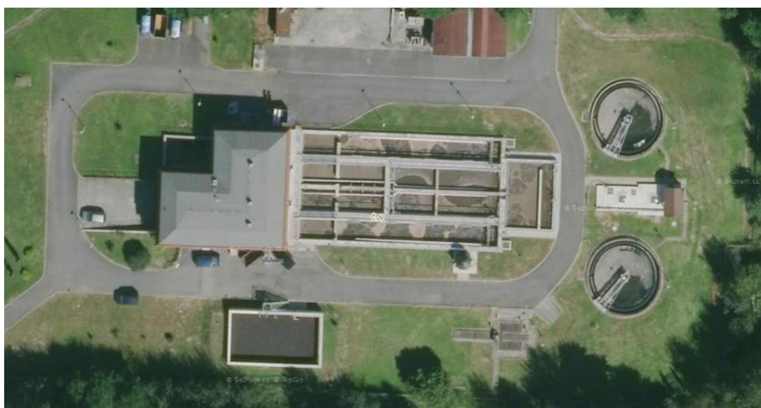
Obr. 27: Letecký pohled na uspořádání dnešní ČOV Tlučná (dostupné z: www.mapy.cz )
