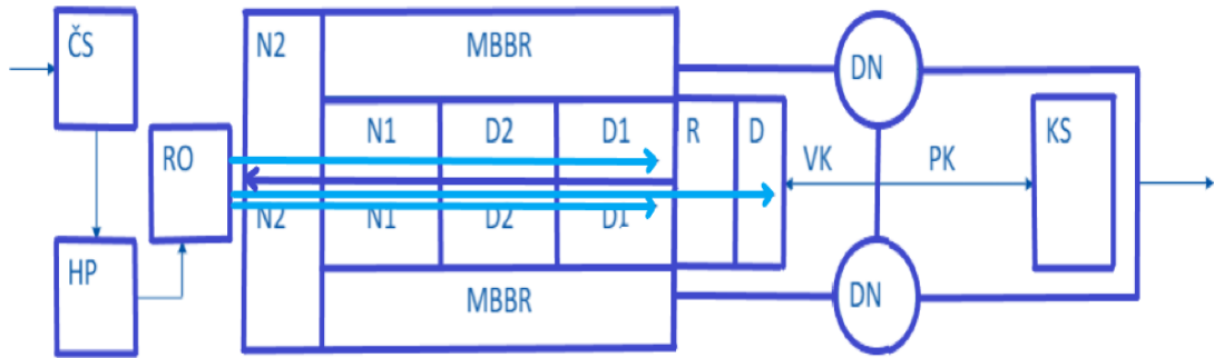
Obr. 29: Zjednodušené schéma ČOV Tlučná po I. intenzifikaci (vlastní nákres)
