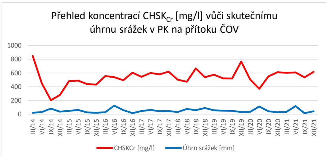
Obr. 46: Přehled koncentrací CHSK Cr [mg/l] vůči skutečnému úhrnu srážek v PK na přítoku ČOV Tlučná (VODÁRNA PLZEŇ a.s., 2022)
