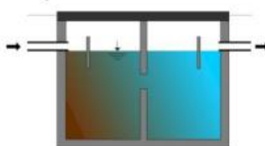
Obr 20: Septik (vlastní nákres)
