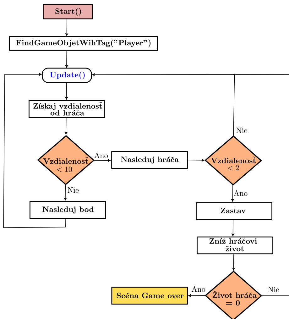
Obrázek 6.29: Algoritmus pohybu ducha po labyrinte. Na začiatku si algoritmus vyhledá hráča. Následne každý snímok sleduje, aká je vzdialenosť medzi duchom a hráčom. Pokiaľ je vzdialenosť menšia ako 10, duch začne hráča prenasledovať až kým sa hráč znovu nevzdiali. Pokiaľ vzdialenosť medzi ním a hráčom dosiahne hodnoty 2, duch zastaví a začne útočiť na hráča. Hráčovi sa začne znižovať úroveň života. Ak hodnota hráčovho života klesne na 0, načíta sa GameOver scéna a hra je ukončená.
