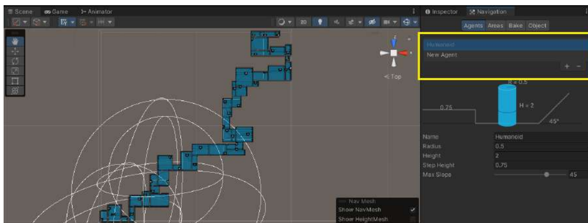
Obrázek 6.23: Aby sa nepriatelia mohli pohybovať po ploche, je potrebné vytvoriť navigačnú sieť. Existujú dva typy sietí – Humanoid a New Agent (žltý rámček). Plochy, na ktorých je NavMesh vytvorený, sú v Unity Editore vyznačené modrou farbou.
