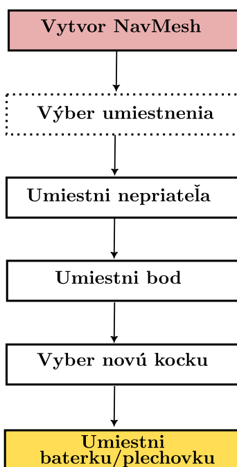
Obrázek 6.24: Algoritmus umiestnenia nepriateľov do labyrintu. Ako prvé algoritmus vytvorí na plochách, kde sa môže nepriateľ pohybovať NavMesh . Keď je vytvorený, môže sa vybrať miesto, kde sa nepriateľ umiestni a následne sa môže na to miesto umiestniť. Spolu s nepriateľom sa umiestni aj bod, ktorý bude prenasledovať. Keď je nepriateľ aj s bodom umiestnený, vyberie sa v rámci izby nová kocka, kam sa umiestni plechovka a baterka.
