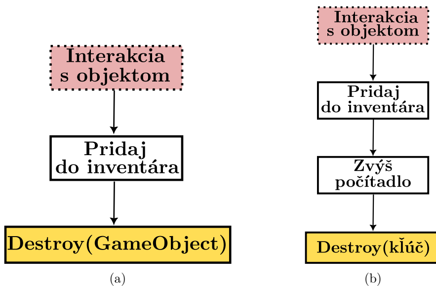
Obrázek 6.41: Obrázky znázorňujú algoritmus zdvihnutia predmetov zo zeme. V prípade zbierania predmetov sa hráčovi po stlačení "E" pridá objekt do inventára a fyzicky je odstránený z hernej scény. V prípade kľúčov, dôjde aj k zvýšeniu počítadla, čím sa aj hráčovi zmení informácia o počte kľúčov na obrazovke (obrázok b).
