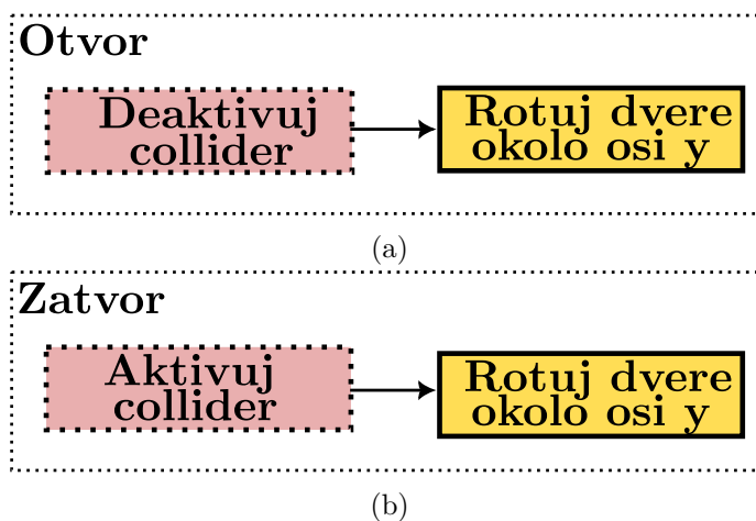
Obrázek 6.44: Dvere rotujú okolo osi y. V prípade otvárania dverí sa ich pozícia posunie v smere osi y o -2, v prípade zatvorenia o 2. Predtým, než sa dvere otvoria (obrázok a) sa deaktivuje kocka, ktorá slúži ako zábrana, aby mohol hráč prejsť cez dvere. V prípade zatvorenia sa táto kocka znovu aktivuje
