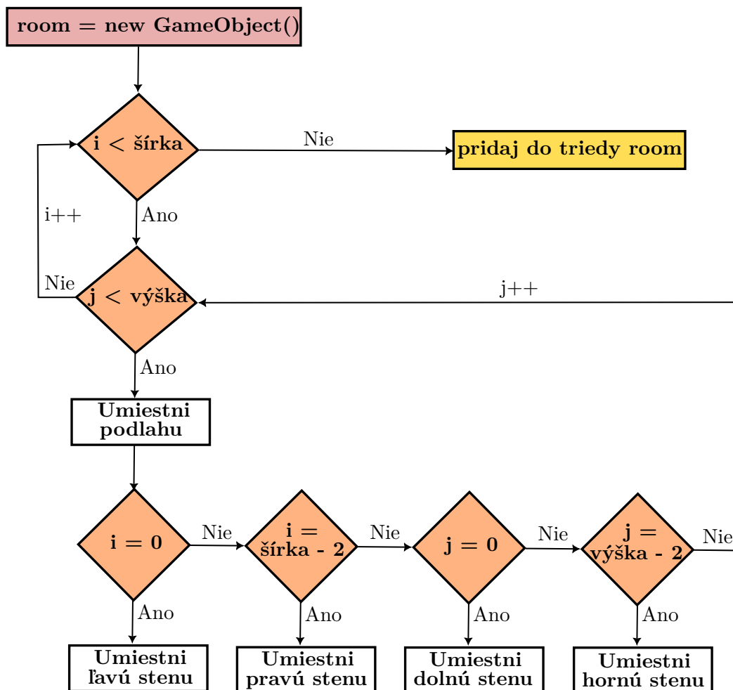
Obrázek 6.15: Obrázok zobrazuje algoritmus, ktorým sa vytvárajú jednotlivé miestnosti. Miestnosť nie je žiadnym statickým objektom, ale dynamicky sa pre každú novú miestnosť vytvára nový GameObject room . Po vytvorení tohto objektu sa iteratívne prechádza cez každý riadok a stĺpec miestnosti. Podľa aktuálnej polohy v mriežke sa kocka (prefab) umiestni na príslušné miesto. Keď je izba vytvorená pridá sa do zoznamu vytvorených izieb.
