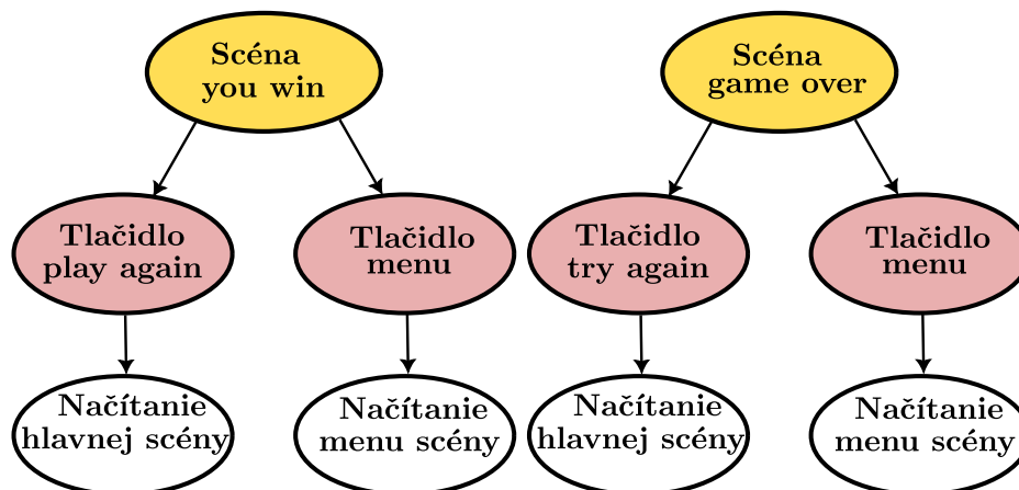
Obrázek 6.4: Scény You win a Game over obsahujú len dve tlačidlá – jedno na načítanie hlavnej hernej scény Main a druhé, ktorým je možné sa vrátiť do Menu .
