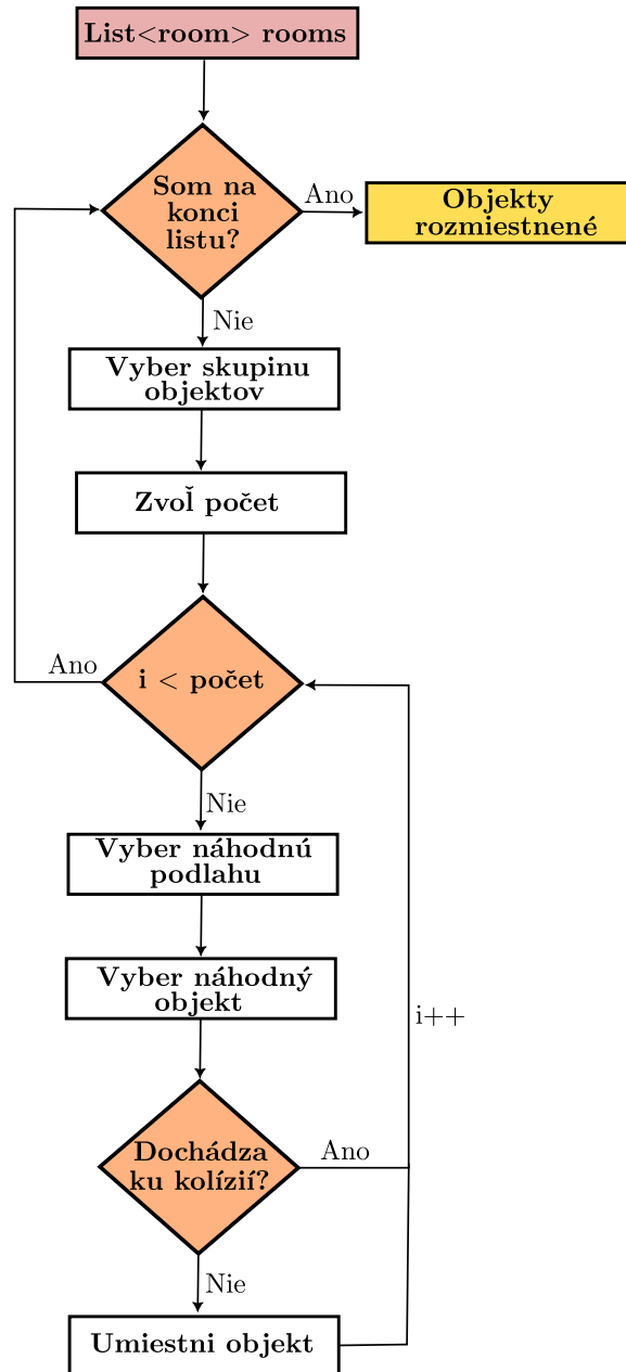
Obrázok 6.20: Obrázok znázorňuje algoritmus, ktorý rozmiestňuje jednotlivé objekty po labyrinte. Algoritmus, na rozdiel od ostatných, nevyberá náhodnú izbu ale postupne prechádza izbu po izbu a umiestňuje do nich objekty. Jednotlivé objekty sú rozdelené do 4 skupín – obývačka, kuchyňa, spálňa a kúpeľňa. Z tejto skupiny sa náhodne zvolí jedna. Následne sa zvolí náhodný počet objektov, ktoré sa budú do miestnosti generovať. Cyklicky sa prechádza týmto počtom a zakaždým sa zo skupiny vyberie náhodne jeden objekt, ktorý sa umiestní na náhodne vybranú podlahu v miestnosti. Pred umiestnením objektu dochádza najskôr ku kontrole, či v mieste umiestnenia nedochádza ku kolízií s iným objektom, prípadne stenou. Ak áno, objekt v tom prípade umiestnený nebude.
