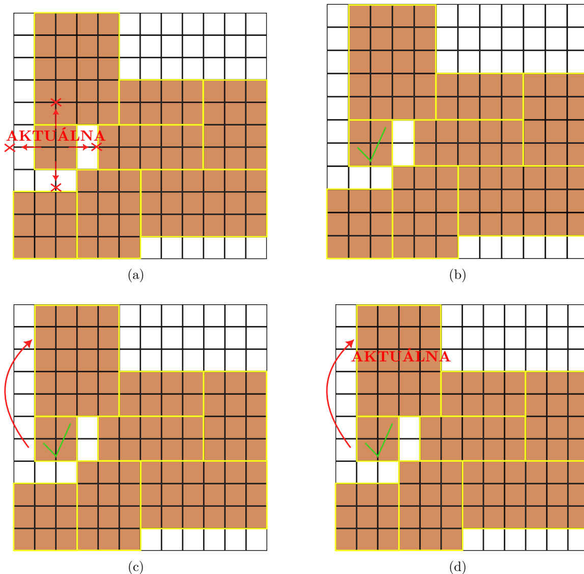
Obrázok 4.6: Princíp backtrackingu pri umiestňovaní izieb. Okolo aktuálne spracovávanej izby nie je žiadny priestor, kde by sa mohla vytvoriť nová izba (obrázok a). Izba sa preto označí ako spracovaná (obrázok b). Algoritmus sa posunie na predchádzajúcu izbu (obrázok c). Tá sa stane aktuálnou a algoritmus sa pokúsi novú izbu vygenerovať vedľa nej (obrázok d).
