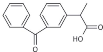
Obrázek 5 - Chemická struktura ketoprofenu (Tuchiu et al. 2022).
