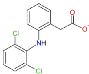
Obrázek 2 - Chemická struktura aniontu diklofenaku (Reyes-García et al. 2021).
