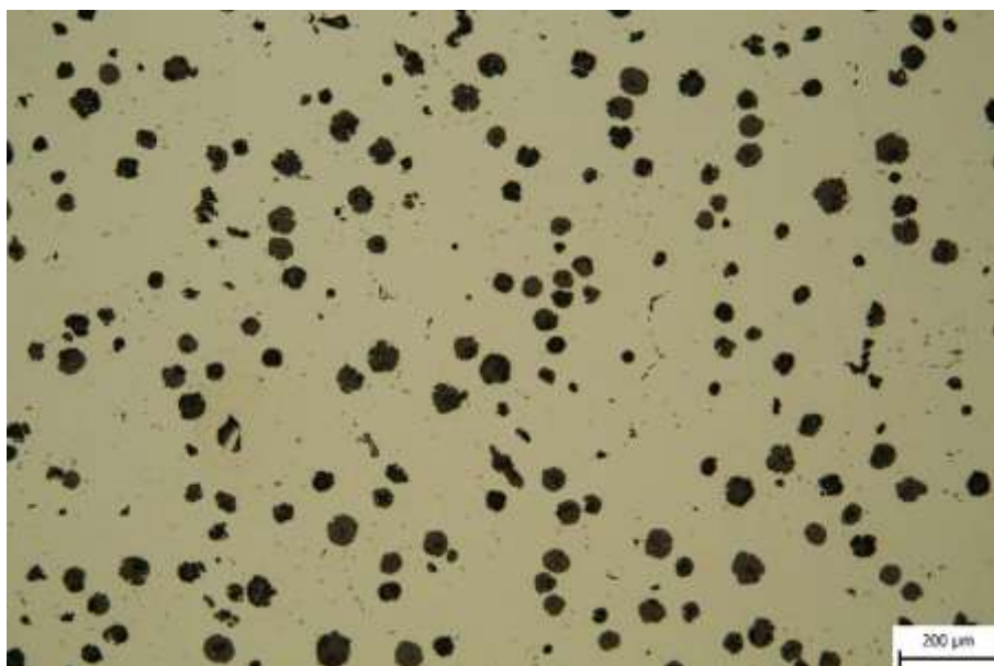
Obr. 69 Výbrus T3-Y100-M3 pořizený 50 od stěny odlitku Y100. Původní zvětšení: 100x.
