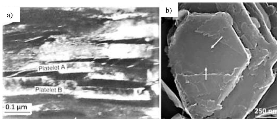
Obr. 9 Vzhled vrstev grafitu a) TEM snímek vrstev grafitu v kuličkovém útvaru grafitu. b) SEM snímek růstové fronty nové destičky grafenu na útvaru vermikálního grafitu. [25].
