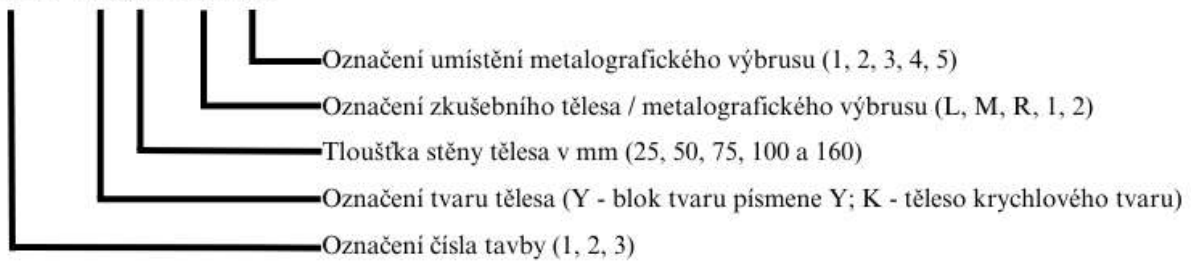
Obr. 37 Systém značení odlitků, těles pro tahovou zkoušku a metalografických výbrusů.
