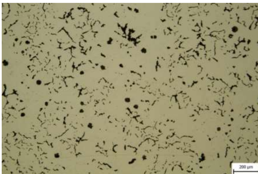
Obr. 63 Výbrus T1-Y100-M1 odpovídající tělesu T1-Y100-L. Původní zvětšení: 100x.
