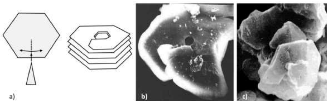
Obr. 14 Šroubovicový růst grafitu s negativním úhlem; a) Schématické znázornění; b) Překrývající se segmenty s dírou hexagonálního tvaru uprostřed; c) Detail na útvar chunky grafitu v LKG [1].
