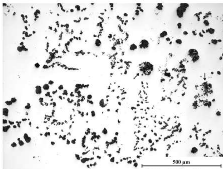
Obr. 34: Mikrostruktura obsahující chunky i explodovaný (označeno šipkami) grafit [57].
