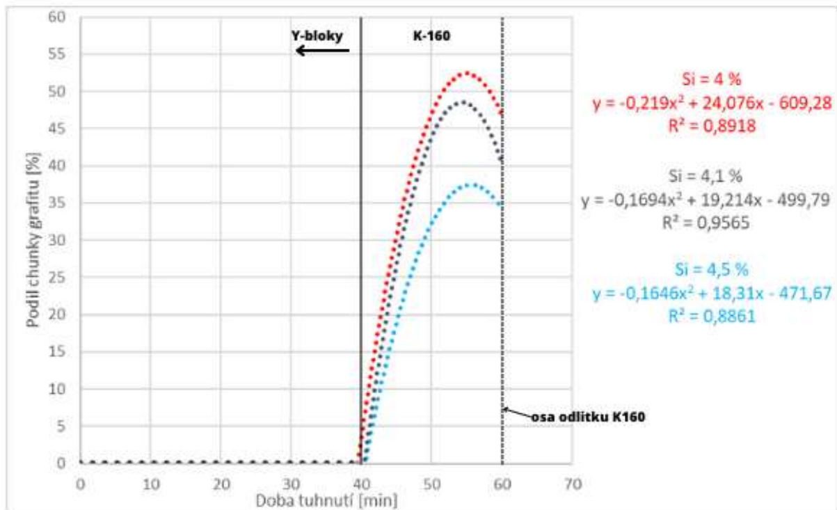
Obr. 79 Závislost podílu chunky grafitu na rychlosti ochlazování pro všechny tvavky.
