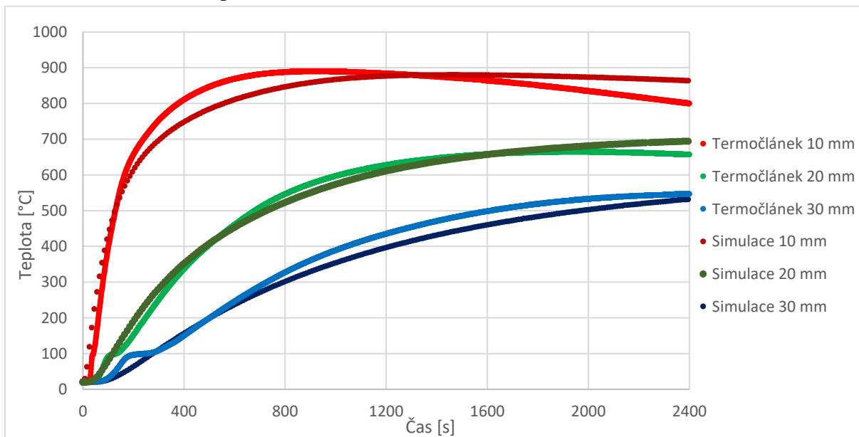
Obr. 42 Graf znázorňující teploty písku v závislosti na čase.
