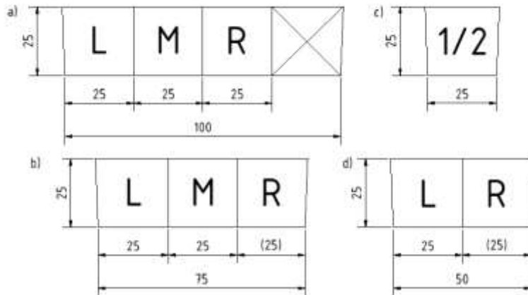
Obr. 38 Schéma značení zkušebních těles pro tahovou zkoušku; a) Y100; b) Y75; c) Y25; d) Y50.
