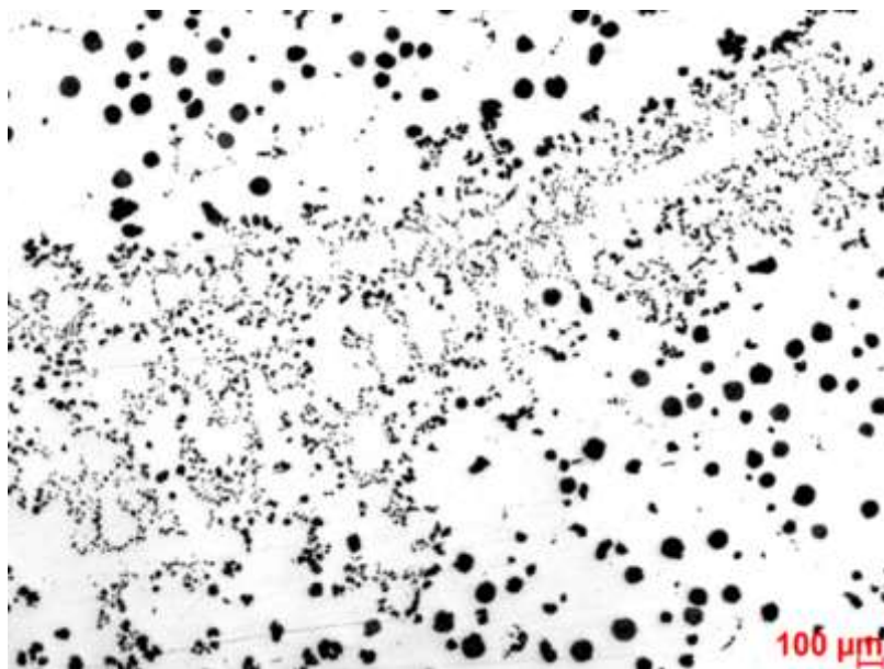
Obr. 1 Mikrostruktura litiny s kuličkovým grafitem se zvýšeným obsahem křemíku obsahující chunky grafit. Původní zvětšení: 50x.
