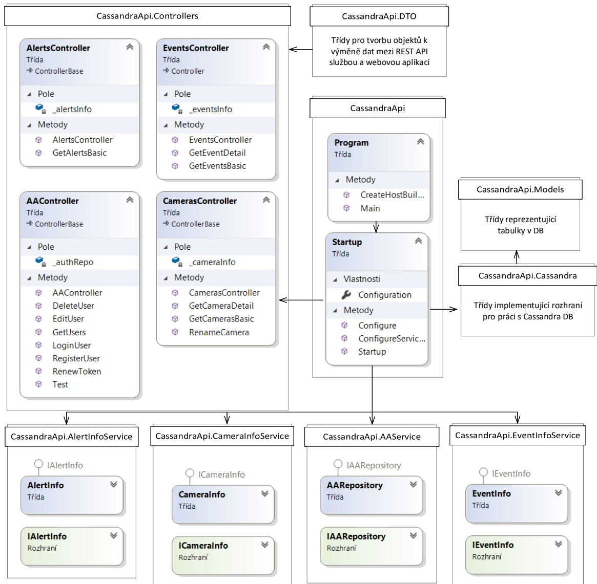
Obr. 2.7: Zjednodušený diagram tříd REST API služby.
