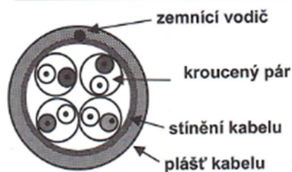
STP/FTP - celkově stíněný párový kabel
