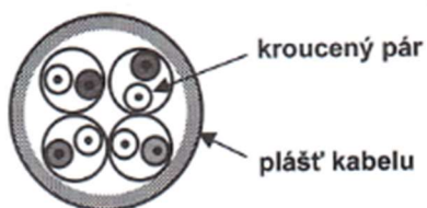
ISTP - celkově stíněný párový kabel se stíněním jednotlivých párů
