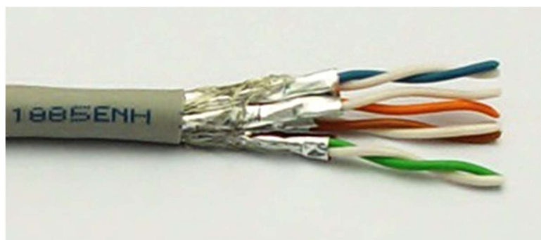
Obrázek 12: příklad kabelu se stíněním jednotlivých párů (Zdroj: 9)
