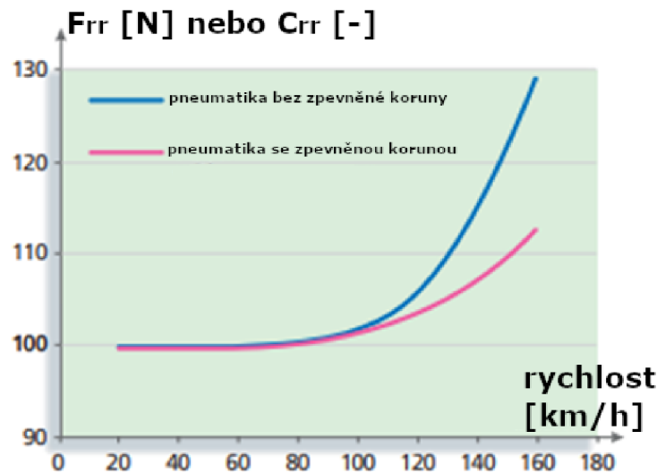
Obrázek 15 Závislost valivého odporu na rychlosti pro automobilové pneumatiky [1] (upraveno)
