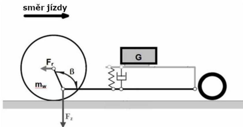
Obrázek 36 Schéma měřicího přivěsu využívající měření pomocí ramena [59] (upraveno)
