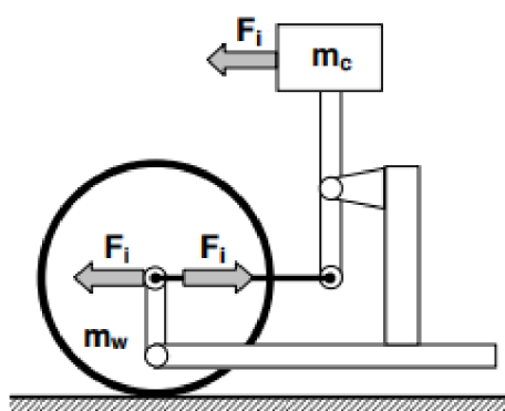
Obrázek 37 Schéma měřicího přívěsu s přidáním kompenzačním členem [59]
