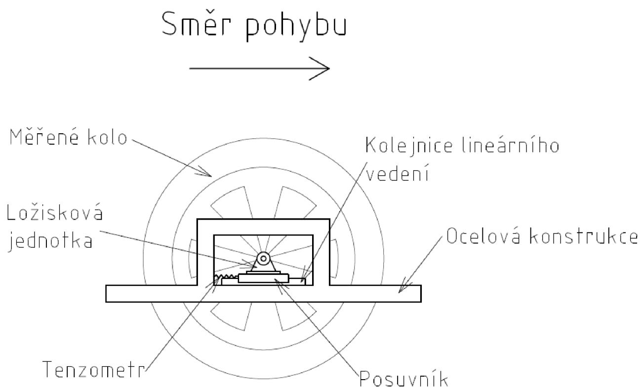
Obrázek 46 Schéma ocelové konstrukce s měřicími prvky
