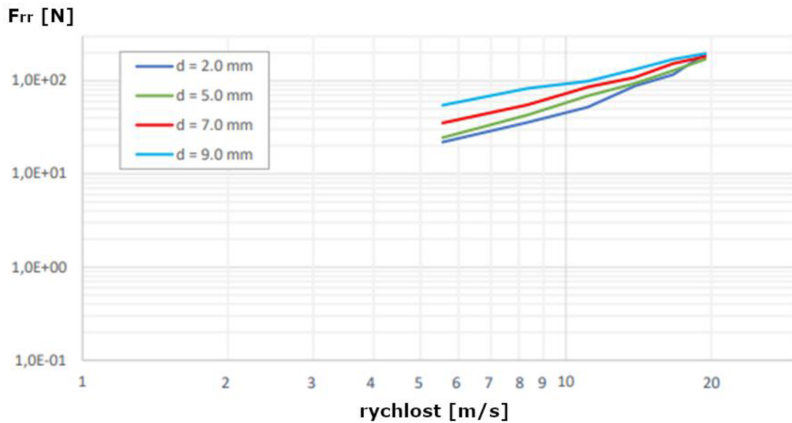
Obrázek 20 Vliv výšky vody na vozovce na valivý odpor [35] (upraveno)
