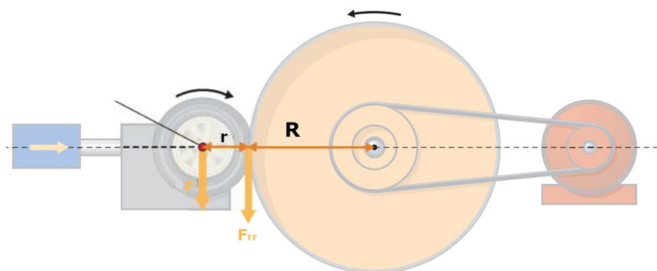
Obrázek 27 Měření na bubnové zkušební pomoci silové metody [1] (upraveno)
