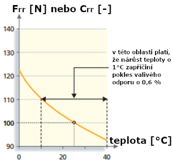
Obrázek 13 Závislost valivého odporu na teplotě pro automobilové pneumatiky [1] (upraveno)
