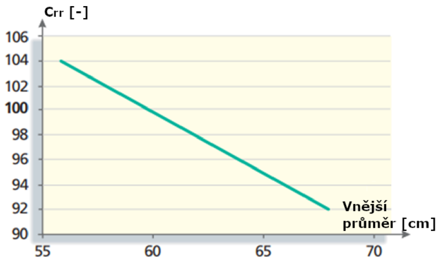
Obrázek 10 Závislost koeficientu valivého odporu na průměru kola [1]
