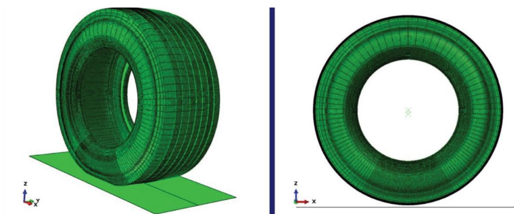
Obrázek 35 Model pneumatiky se sítí konečných prvků [58]
