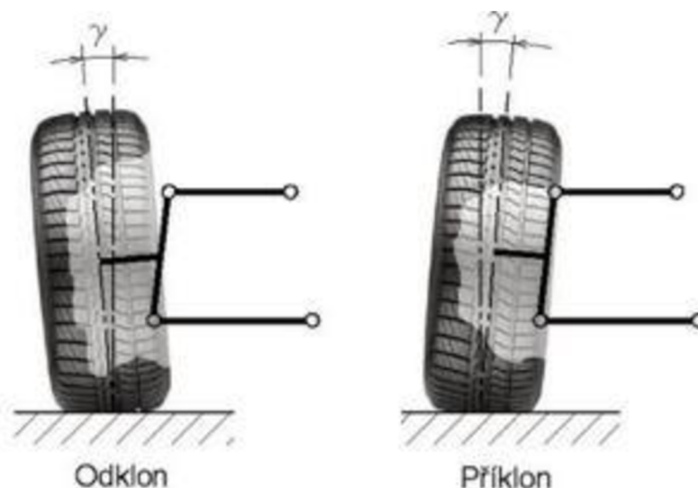
Obrázek 24 Znárodnění úhlu odklonu a příklonu kola [44]
