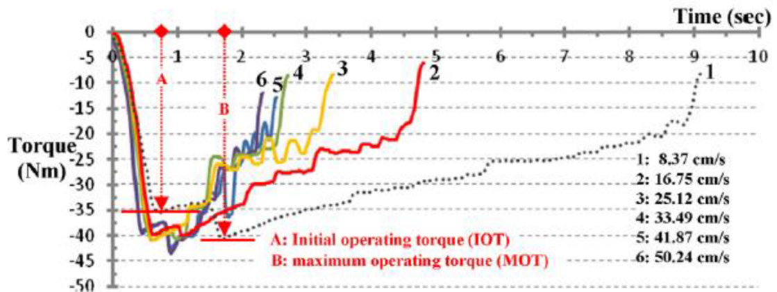
Obrázek 6.4 - Měření momentu síly k ose pro dveře se zavíračem určeným pro těžké dveře [30]
