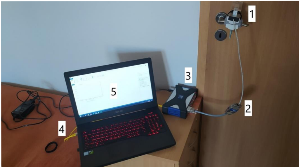
Obrázek 3.9 - Celkové zapojení měřicího řetězce
