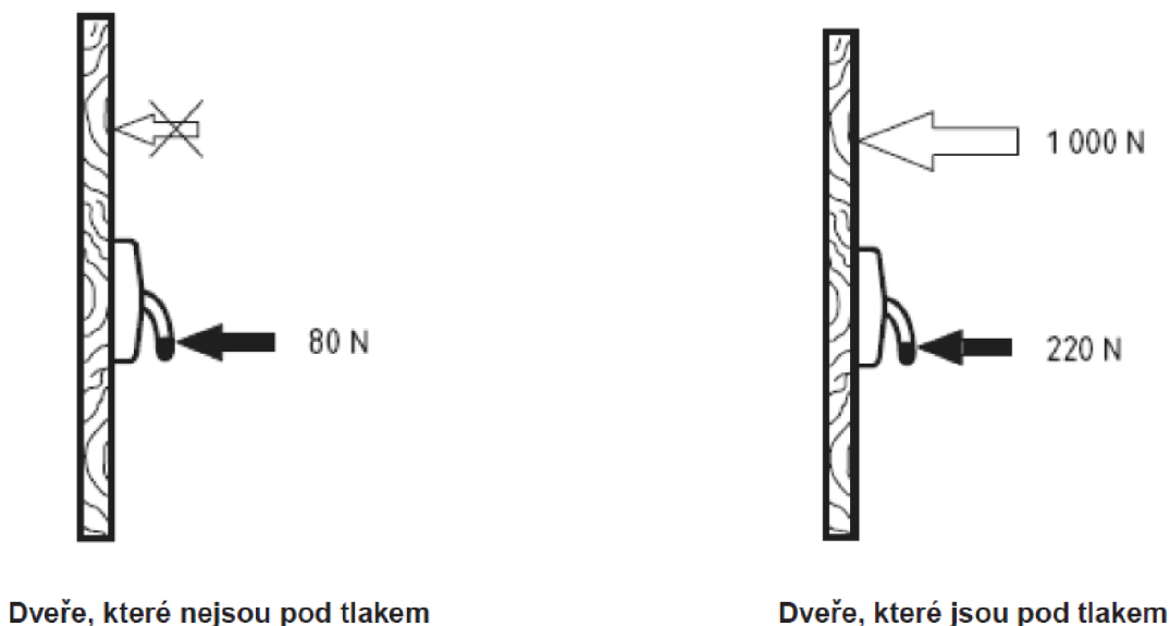
Obrázek 2.4 - Uvolňovací síly panikových dveřních uzávěrů dle normy ČSN EN 1125 [8]
