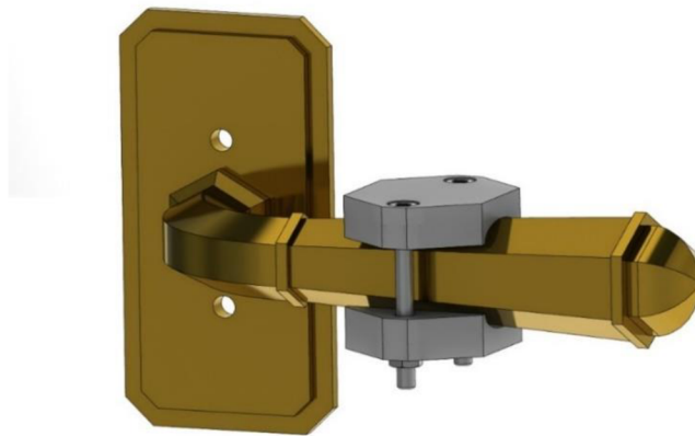
Obrázek 3.4 - Druhý model úchytu na kliku umístěný na klice
