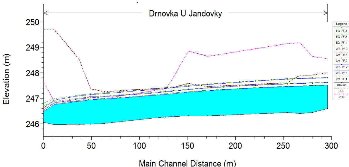
Obr. 5.7 Podélný profil toku Drnovka
