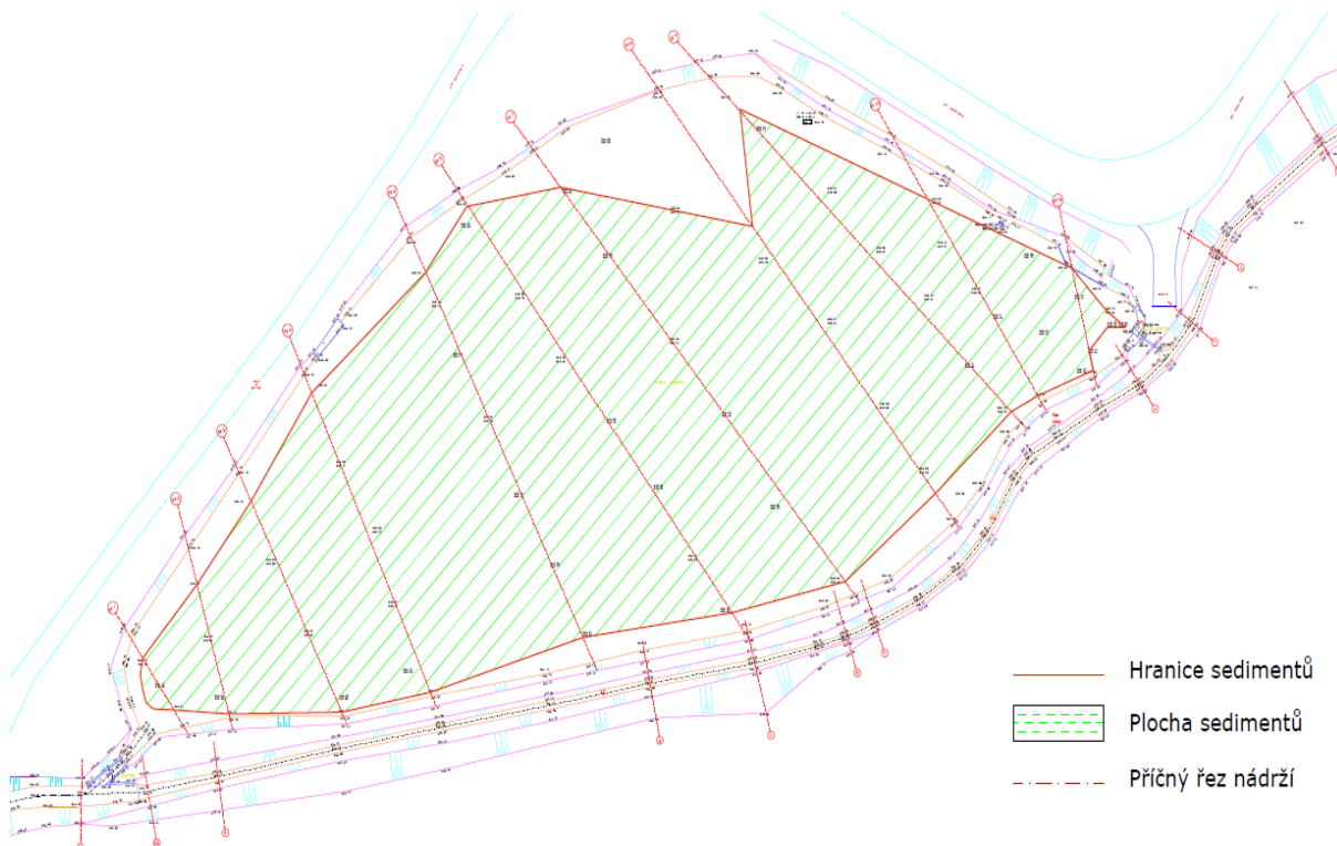
Obr. 5.1 Schématické znázornění plochy sedimentů v nádrži
