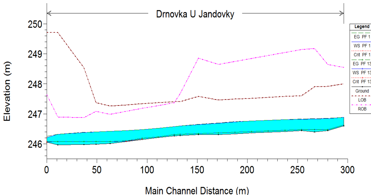
Obr. 5.5 Podélný profil toku Drnovka pro Q_m
