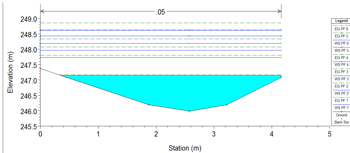
Obr. 5.3. Příčný profily toku Drnůvka, PF5 0,063 km
