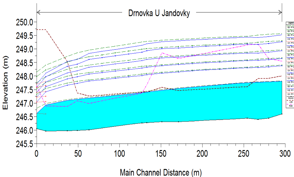
Obr. 5.4. Podélný profil toku Drnůvka pro Q_N
