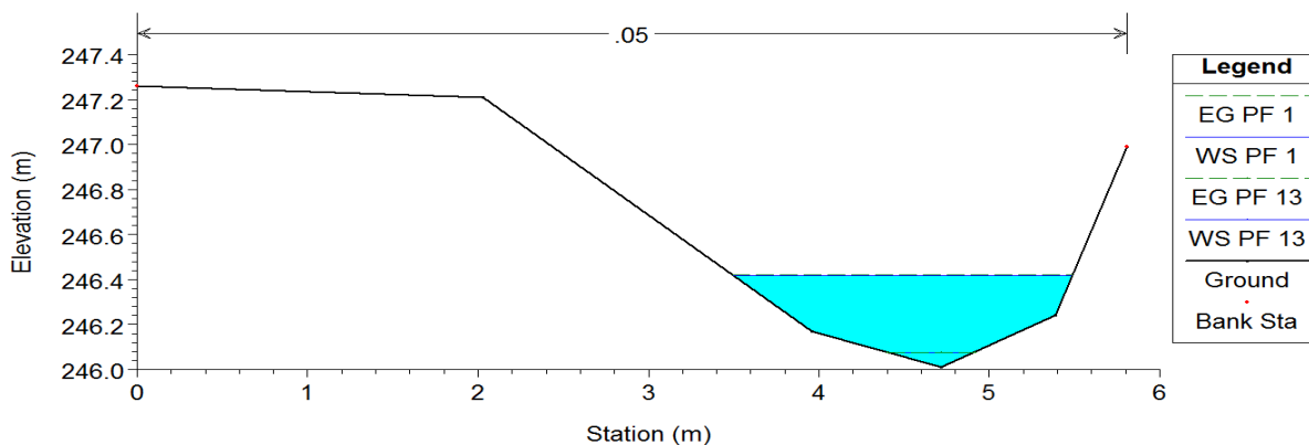
Obr. 5.6 Příčný profil toku Drnovka, PF5 0,063 km
