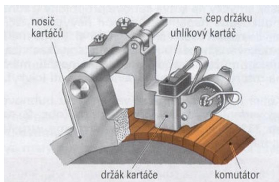
Obr.2.1 Komutátor [7]
