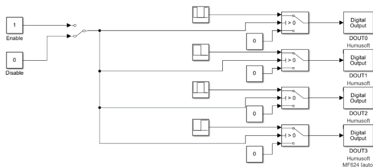
Obr. 3.17. Ukázka nejjednoduššího ovládání krokového motoru
