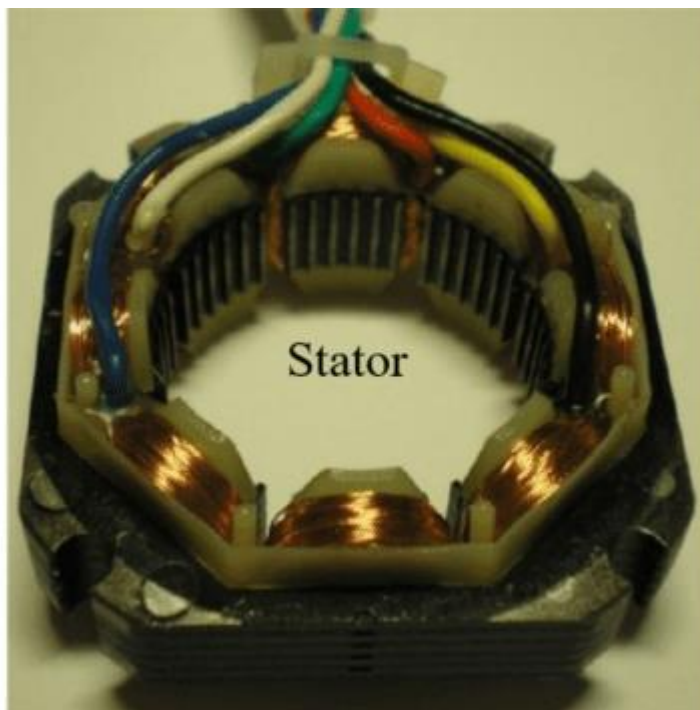
Obr.2.7 Cívky statoru [5]
