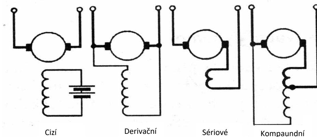
Obr. 2.4 Možná zapojení buzení motoru [13]
