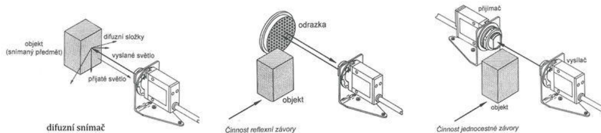
Obr.2.15. Typy optických závor [9]
