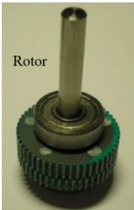
Obr.2.6 Vzájemně posunuté magnety [5]
