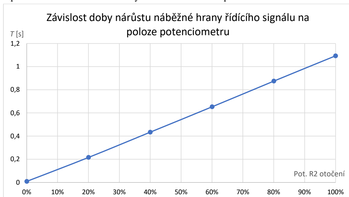
Obrázek 20: Závislost doby nárůstu náběžné hrany řídicího signálu na poloze potenciometru
