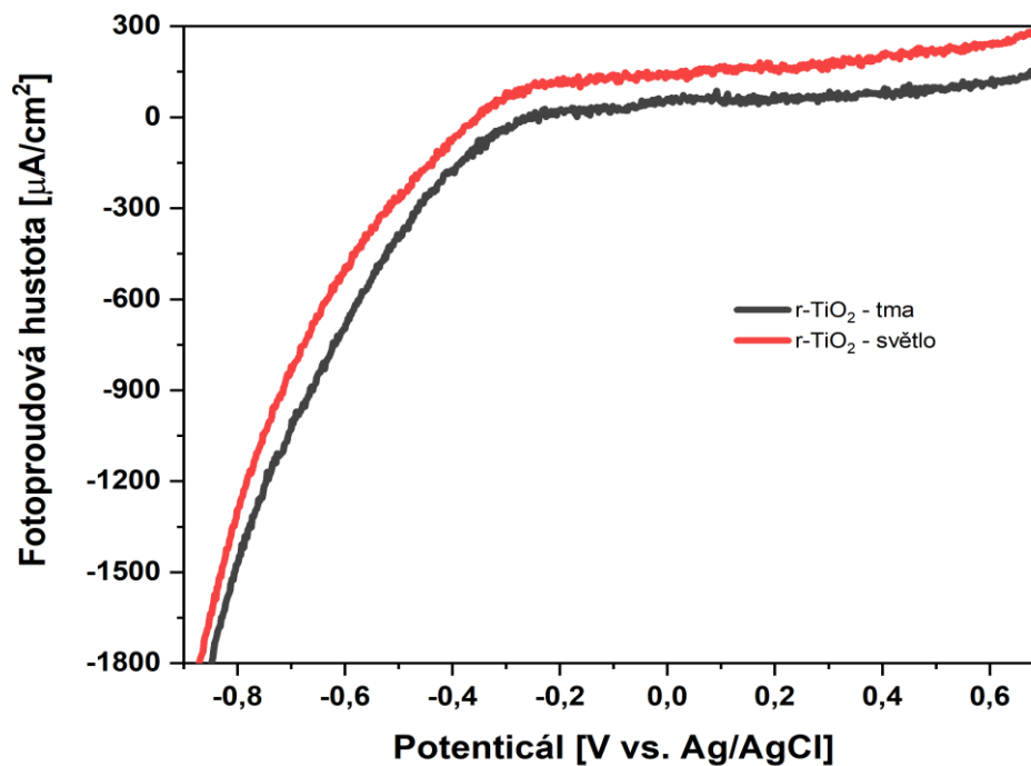
Obrázek 27: Grafická závislost fotoproudové hustoty na vloženém potenciálu proti referenční elektrodě pro vzorky nanotubic r-TiO 2 .
