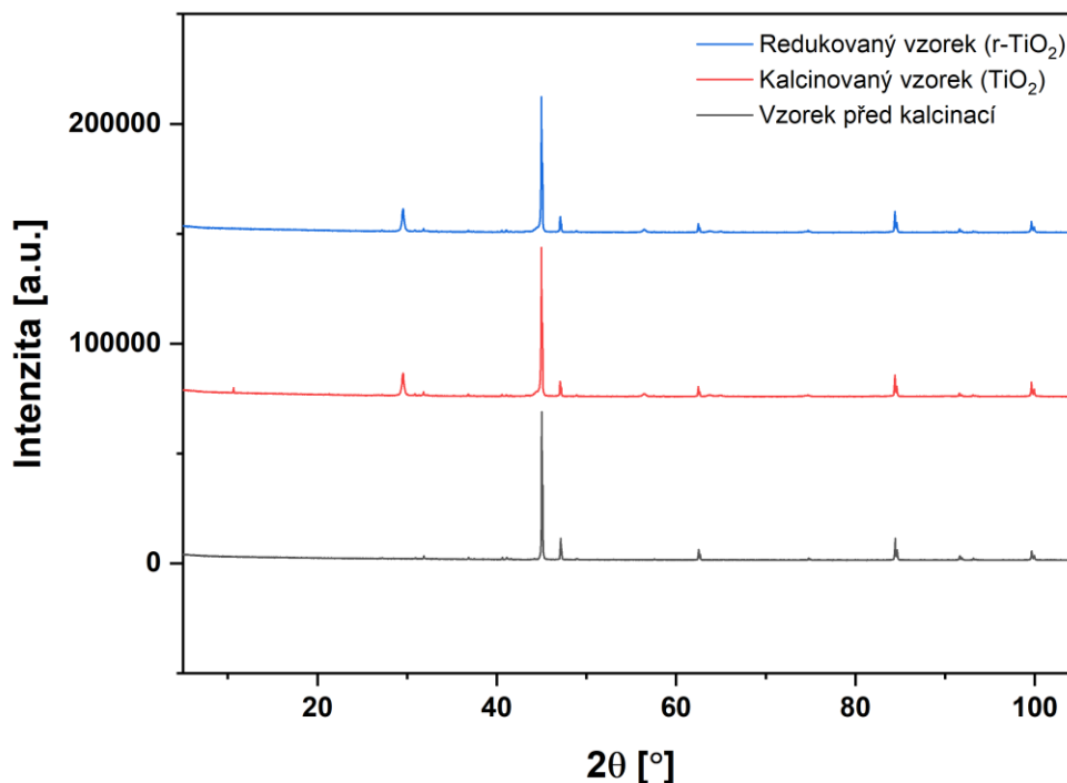
Obrázek 23: XRD difraktogram pro vzorek před kalcinací, po kalcinaci a redukovaný vzorek.
