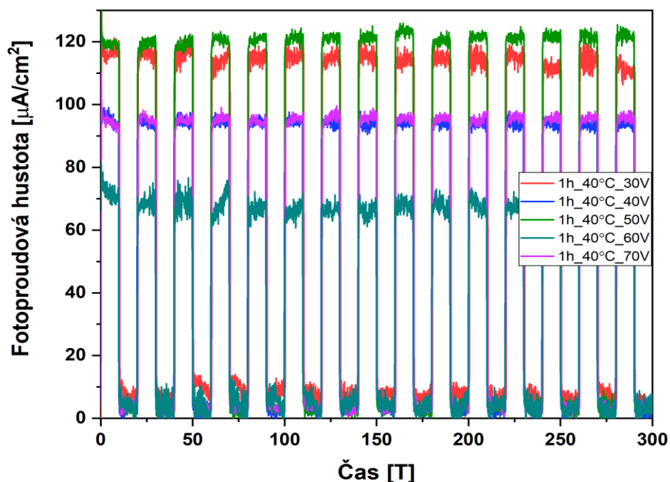
Obrázek 30: Grafická závislost fotoproudové hustoty na čase měření pro vzorky nanotrubic \text{TiO}_2 připravených při 1 hodině, 40^\circ\text{C} a různém napětí vloženém na elektrody.
