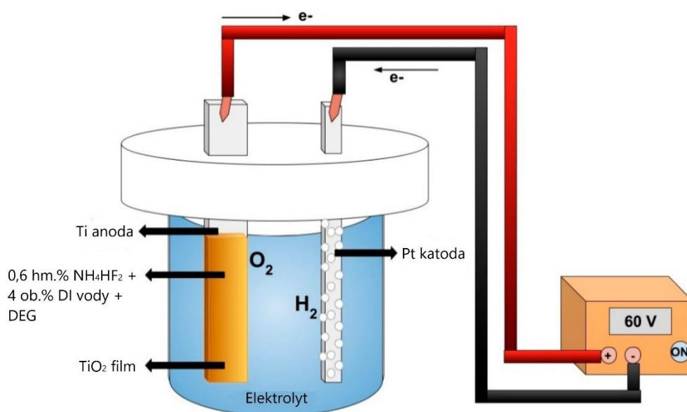
Obrázek 6: Schematicky znázorněna příprava nanotubic TiO 2 elektrochemickou anodizací. Převzato a upraveno z [43].
