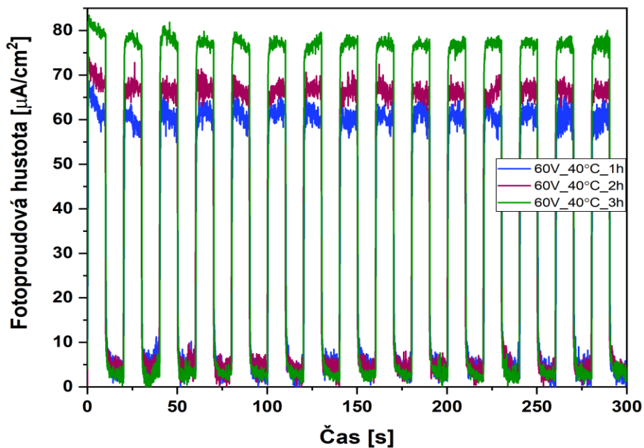
Obrázek 32: Grafická závislost fotoproudové hustoty na čase měření pro vzorky nanotrubic \text{TiO}_2 připravených při 60 V, 40 °C a různém čase.
