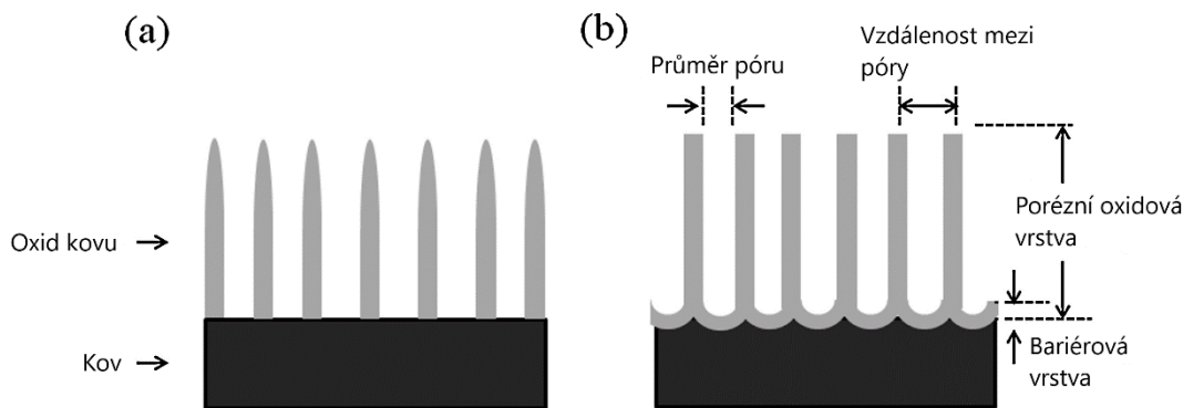
Obrázek 4: a) Pozitivní templát – vznikající nanotrubice rostou na povrchu templátu. b) Negativní templát – vznikající nanotrubice rostou uvnitř pórů templátu. Převzato a upraveno z [23].
