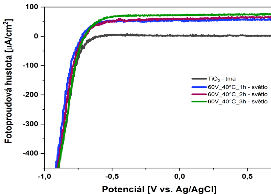
Obrázek 31: Grafická závislost fotoproudové hustoty na vloženém potenciálu proti referentní elektrodě pro vzorky nanotrubic \text{TiO}_2 připravených při 60 V, 40 °C a různém čase.
