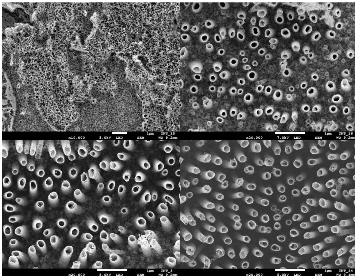
Obrázek 21: SEM snímky čtyř různých vzorků připravených při stejné anodizační době (1 hodina) a vloženém napětí na elektrody ( U = 60 V). Příprava probíhala za různých teplot: a) T = 20 °C, b) T = 30 °C, c) T = 40 °C a d) T = 50 °C.
