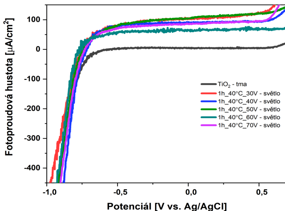
Obrázek 29: Grafická závislost fotoproudové hustoty na vloženém potenciálu proti referenční elektrodě pro vzorky nanotrubic TiO 2 připravených při 1 hodině, 40 °C a různém napětí vloženém na elektrody.
