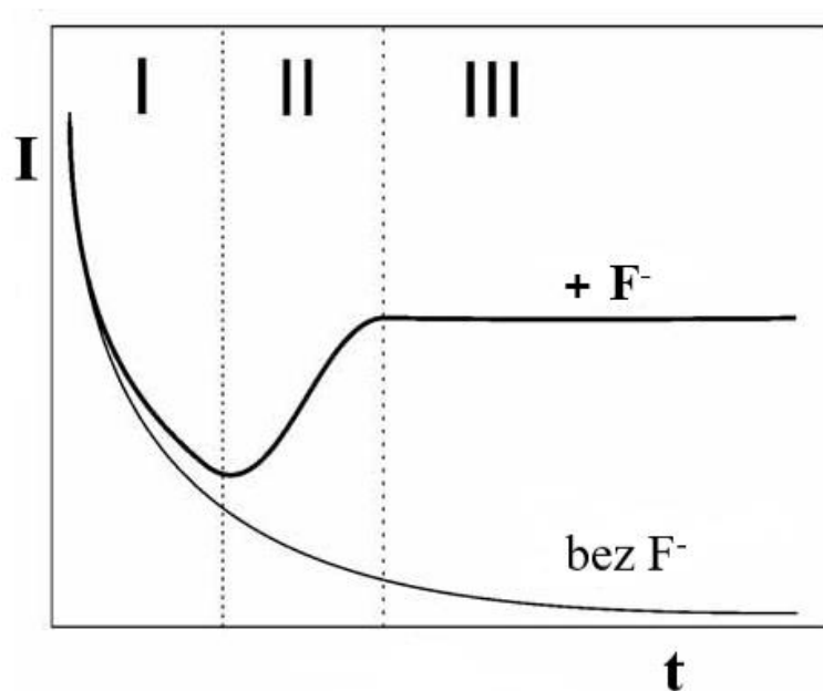
Obrázek 7: Grafické zobrazení závislosti proudu na čase v průběhu elektrochemické anodizace. Tenkou čarou je zobrazen průběh při využití elektrolytu bez obsahu fluoridových iontů. Tučnou čarou je znázorněn průběh popisující tvorbu nanotrubic, tento proces se rozděluje do tří fází. Převzato a upraveno z [47].
