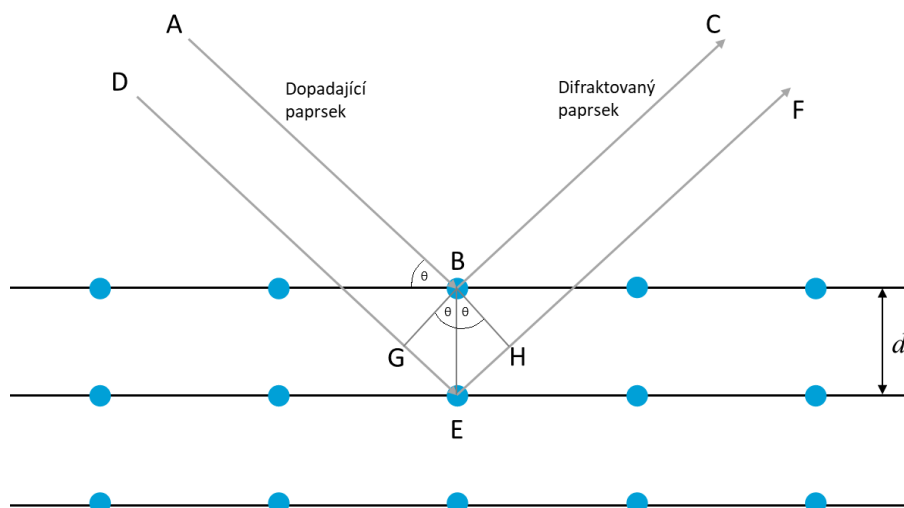
Obrázek 11: Schéma znázorňující difrakci od krystalových rovin na základě Braggova zákona.
