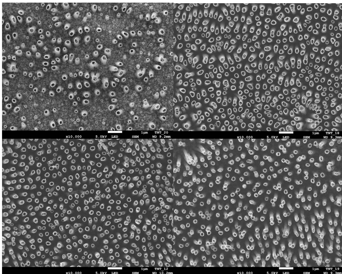
Obrázek 22: SEM snímky čtyř různých vzorků připravených při stejné anodizační době (3 hodiny) a vloženém napětí na elektrody ( U = 60 V). Příprava probíhala za různých teplot: a ) T = 20 °C, b ) T = 30 °C, c ) T = 40 °C a d ) T = 50 °C.
