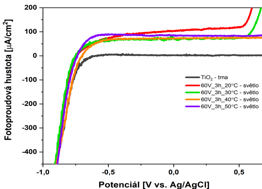
Obrázek 33: Grafická závislost fotoproudové hustoty na vloženém potenciálu proti referenční elektrodě pro vzorky nanotrubic \text{TiO}_2 připravených při napětí 60 V, 3 hodinách a různé teplotě.
