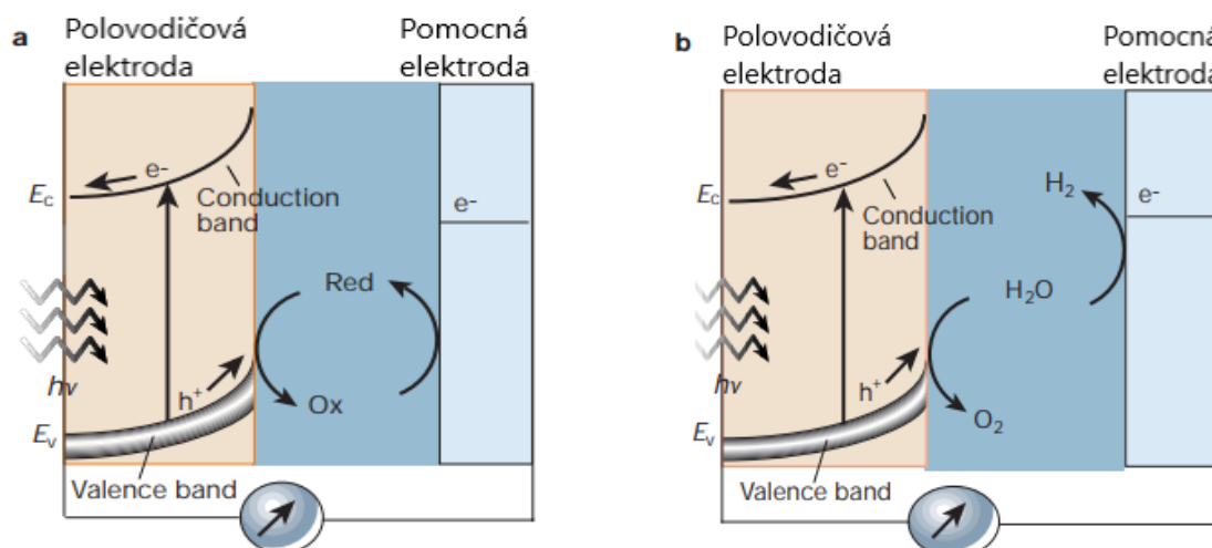
Obrázek 1: Fotoelektrochemické články založené na použití polovodiče typu N jako fotoelektrody. a) Regenerační článek produkující elektrickou energii ze slunečního záření. b) Fotosyntetický článek produkující vodík jako chemické palivo štěpením vody. (Conduction band – vodivostní pás, valence band – valenční pás). Převzato a upraveno z [2].
