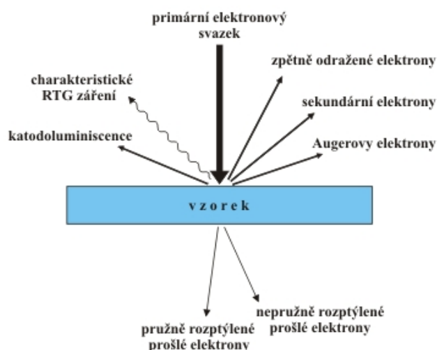
Obr. 6.3: Schéma interakce dopadajícího elektronového svazku s povrchem [43].
