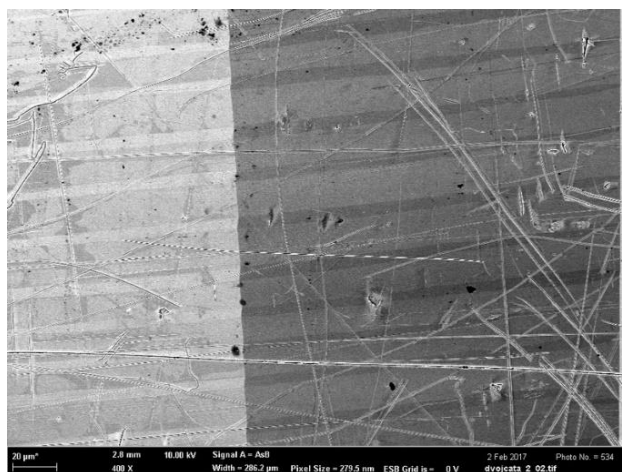
Obr. 7.8: Interakce a/c dvojčatění se složeným dvojčatěním při zvětšení 400x.
