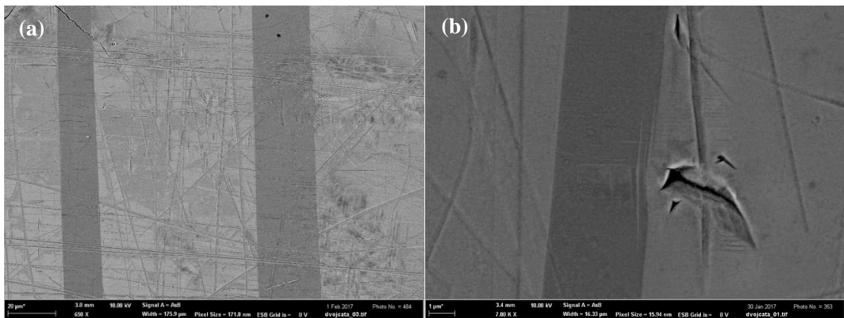
Obr. 7.7: Povrch vzorku pozorovaný pomocí elektronového mikroskopu při zvětšení 650x (a) a interakce hranic dvojčatění s defektem při zvětšení 7000x (b).
