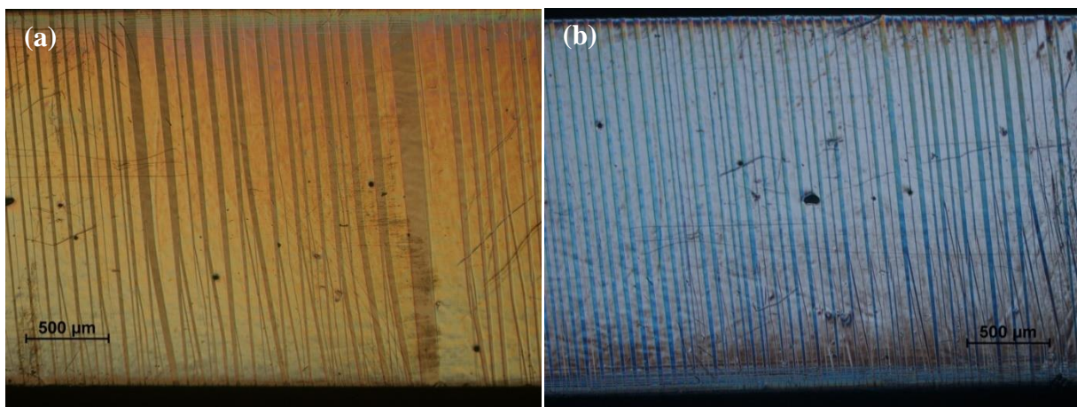
Obr. 7.5: Různá zbarvení struktury obsahující a/c dvojčatění vyvolaná metodou DIC při zvětšení 50x.
