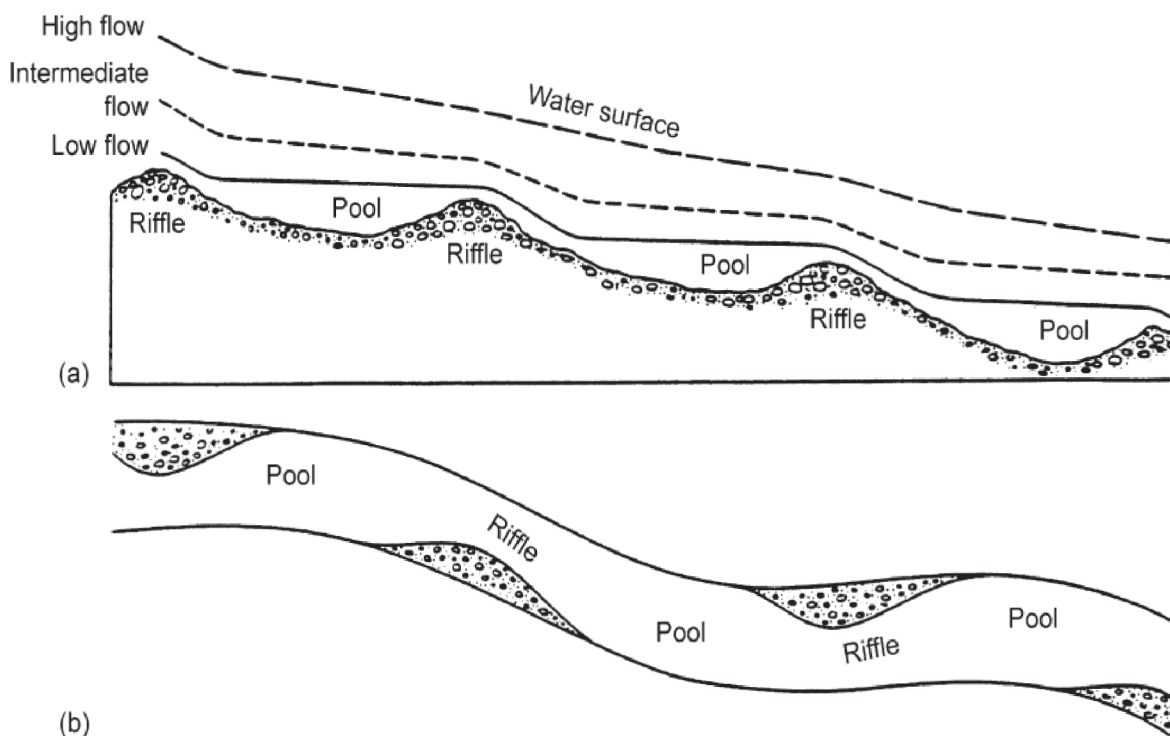
Obrázek 3.1.2 a) Podélný profil s ukázkou střídání tůň – peřej, znázornění podmínek vysokého, středního a nízkého průtoku; b) Pohled shora na sekvenci tůň a peřej (Allan & Castillo, 2007)
