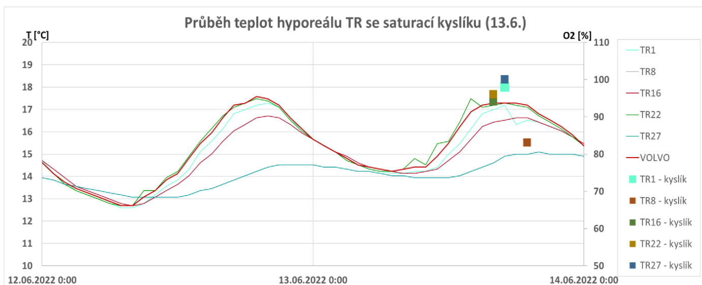
Obrázek 5.2.5 Znárodnění průběhu teplot hyporeálu horních profilů na pěti měrných bodech plochy Transekt (linie). Jedná se o období 12.6.–14.6. 2022. Doplňkově byla měřena saturace kyslíku na totožných pěti bodech (body). Míra okysličení hyporeálu byla měřena 13.6. v rozmezí 16-19 hodiny odpolední (vyznačeno rozestupem). Svislá hlavní osa (vlevo) zobrazuje teplotu (°C). Svislá vedlejší osa (vpravo) zobrazuje procentuální saturaci kyslíku (%O 2 ).
