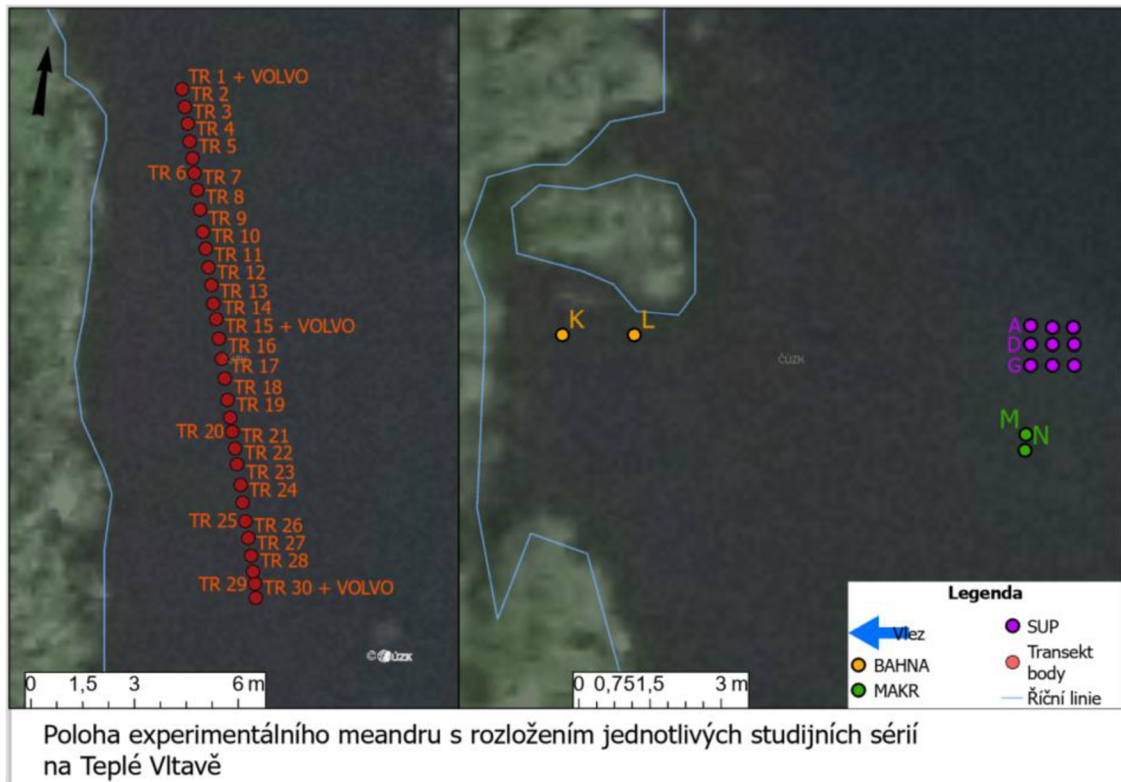
Obrázek 4.2.2 Detailní rozpis umístění čidel v rámci samostatných sérií. Vlevo: podrobný pohled na uložení samostatných teploměrů. VOLVO – čidlo pro měření volně proudící vody. Vpravo: podrobný pohled na uložení samostatných teploměrů dle sérii viz Legenda. SUP – superčtverec; MAKR – makrofyta. Souřadnicový systém S-JTSK (ČUZK, 2023). Zpracováno autorem.
