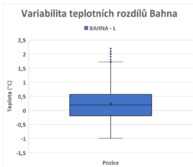
Obrázek 5.5.3 Variabilita rozdílových teplotních údajů mezi horními a dolními hloubkovými profilech. Měřeno na dvou měrných bodech plochy Bahna. Chybová čidla nebyla do grafu zapojena. V případě chyby jednoho z dvojice profilů, nebyla začazena celá sestava (nebyla možnost rozdílu). Jednotlivé boxploty značí konkrétní měrné body v terénu. Jedná se o období 11.5.–21.10.2022. Svislá hlavní osa (vlevo) zobrazuje teplotu (°C). Záporné číslo značí vyšší teplotu spodního čidla.
