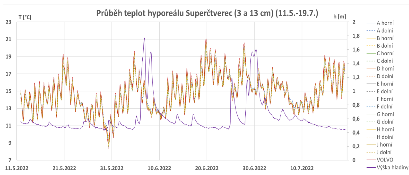
Obrázek 5.3.1 Znárodnění průběhu změny teplot v horních a spodních (3 a 13 cm) hloubkových profilech. Měřeno na devíti měrných bodech plochy Superčtverec. Horní čidlo znázorňuje plná linie, spodní čidlo přerušovaná. Jedná se o období 11.5.-19.7. 2022. Svislá hlavní osa (vlevo) znázorňuje teplotu (°C). Svislá vedlejší osa (vpravo) znázorňuje dynamiku výšky vodní hladiny (m).
