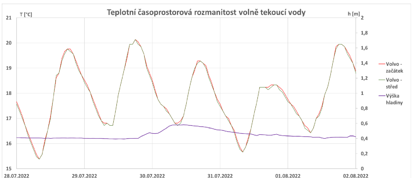
Obrázek 5.1.2 Znárodnění průběhu změn teplot (°C) volně proudící vody z počátku a střední části podélného transektu. Jedná se o výřez z období viz (Obr. 5.1.1.a) od 28.7. do 2.8. 2022. Výřez byl vybrán náhodně za účelem bližší ukázky teplotní oscilace. Svislá hlavní osa (vlevo) znázorňuje teplotu (°C). Svislá vedlejší osa (vpravo) znázorňuje dynamiku výšky vodní hladiny (m).
