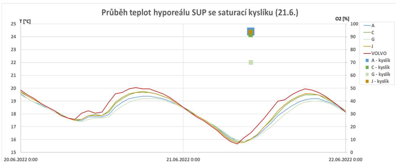
Obrázek 5.3.6 Znáznornění průběhu teplot hyporeálu horních profilů na čtyř měrných bodech plochy Superčtverec (linie). Jedná se o období 20.6.-22.6. 2022. Doplňkově byla měřena saturace kyslíku na totožných čtyřech bodech (body). Míra okysličení hyporeálu byla měřena 21.6. v období krátce po 10 hodině dopolední. Svislá hlavní osa (vlevo) zobrazuje teplotu (°C). Svislá vedlejší osa (vpravo)
