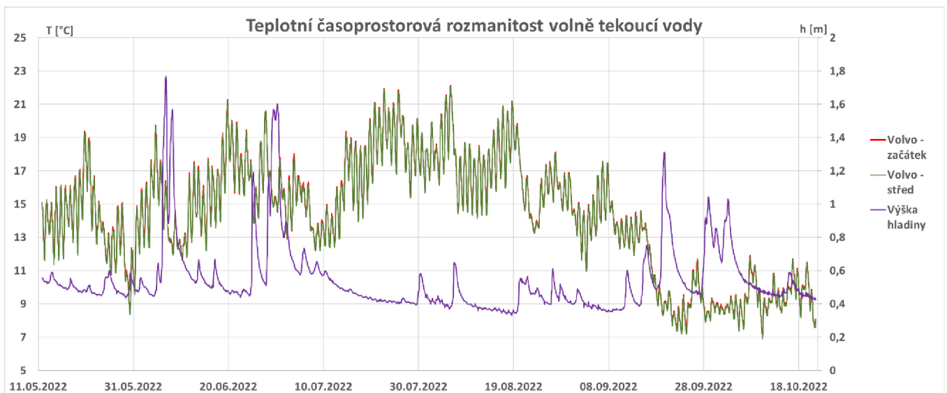
Obrázek 5.1.1 Znárodnění průběhu změn teplot (°C) volně proudící vody z počátku a střední části podélného transektu. Jedná se o časové období od 11.5. do 21.10. 2022. Svislá hlavní osa (vlevo) znázorňuje teplotu (°C). Svislá vedlejší osa (vpravo) znázorňuje dynamiku výšky vodní hladiny (m).
