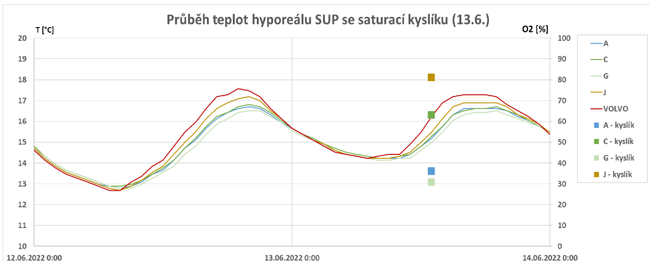
Obrázek 5.3.5 Znáznornění průběhu teplot hyporeálu horních profilů na čtyřech měrných bodech plochy Superčtverec (linie). Jedná se o období 12.6.-14.6. 2022. Doplňkově byla měřena saturace kyslíku na totožných čtyř bodech (body). Míra okysličení hyporeálu byla měřena 13:6. v období od 12 do 13 hodin odpolední. Svislá hlavní osa (vlevo) zobrazuje teplotu (°C). Svislá vedlejší osa (vpravo) zobrazuje procentuální saturaci kyslíku (%O 2 ).
