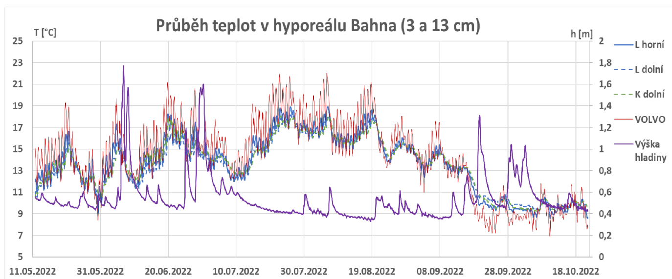
Obrázek 5.5.1 Znárodnění průběhu změn teploty v horních a spodních (3 a 13 cm) hloubkových profilech. Měřeno na dvou měrných bodech plochy Bahna. Chybavá čidla nebyla do grafu zapojena (K horní). Horní čidlo znázorňuje plná linie, spodní čidlo přerušovaná. Jedná se o období 11.5.-21.10.2022. Svislá hlavní osa (vlevo) znázorňuje teplotu (°C). Svislá vedlejší osa (vpravo) znázorňuje dynamiku výšky vodní hladiny (m).
