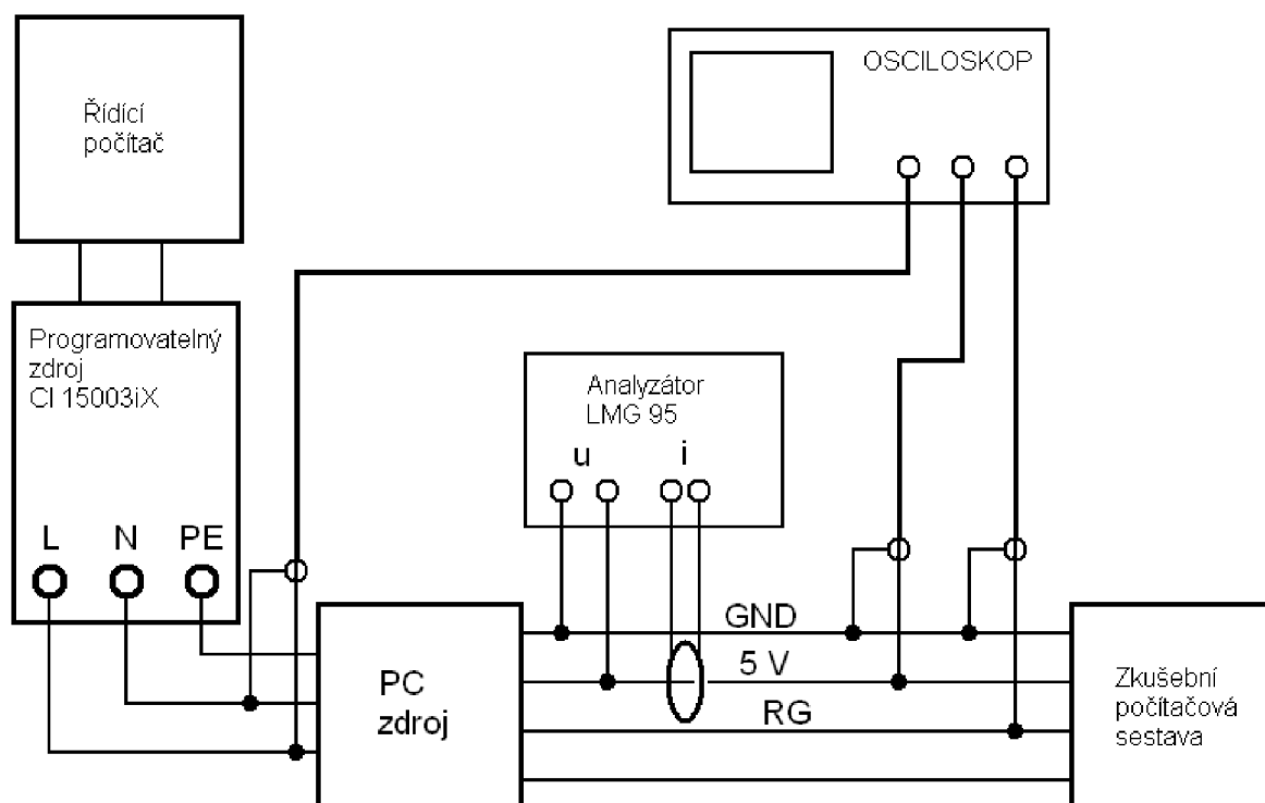
Obr. 6-2 Blokové schéma zapojení měřicích přístrojů
