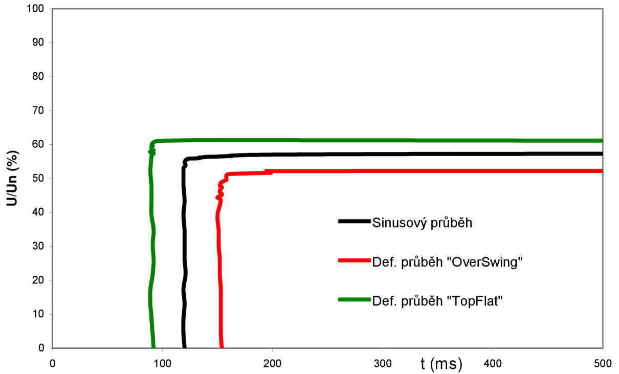
Obr. 7-6 Mezní křivky zdroje FRW 200
