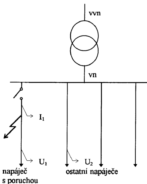
Obr. 2-2 Příklad funkce OZ v rozvodné síti vysokého napětí
