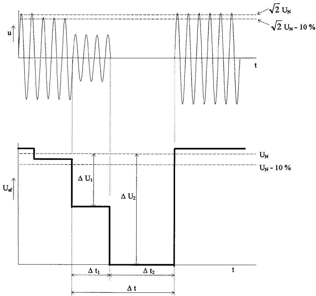
Obr. 2-1 Znáornění poklesu a přerušení napětí
