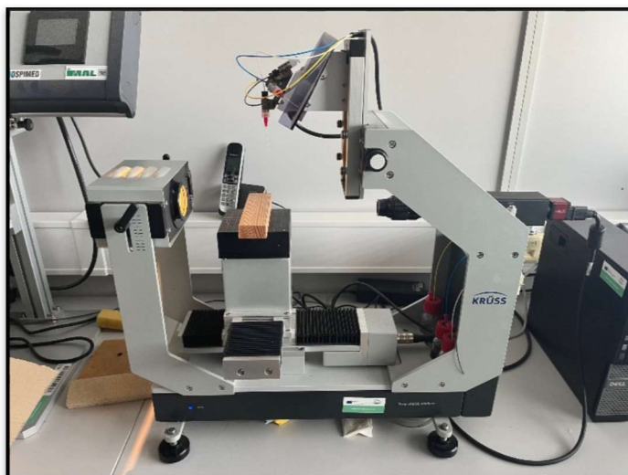
Obr. 24 Meranie zmáčavosti vzoriek pomocou analyzátoru tvaru kvapky KRUSS (zdroj: vlastný)
