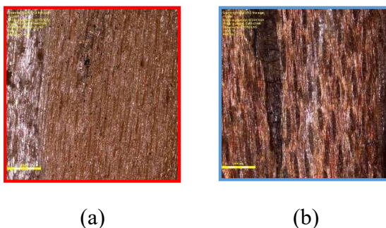
Obr. 26 Mikroskopické zmeny u referenčných vzoriek vystavených v exteriéri po dobu 3 mesiacov. Obrázky zobrazujú: (a) najväčšiu zmenu (MD-REF-2), (b) najmenšiu zmenu (MB-REF-2)
