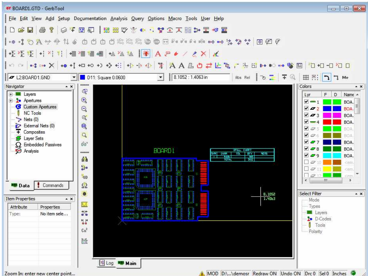
Obr. 3.12 GerbTool
