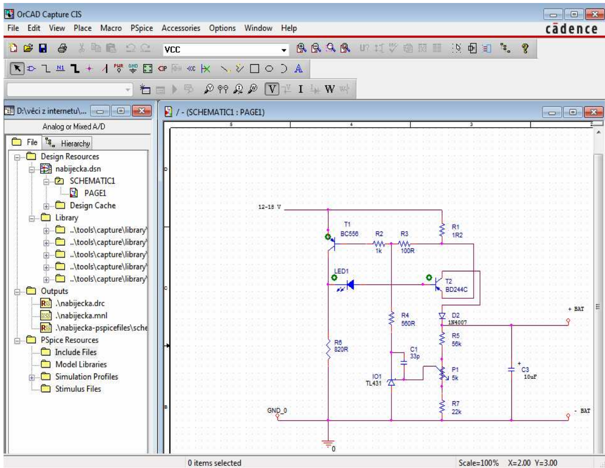
Obr. 3.3 Návrh schématu
