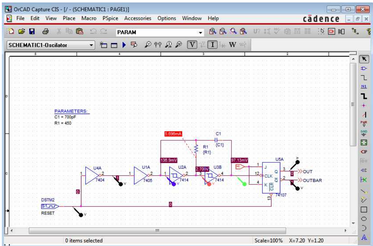
Obr. 4.12 Schéma zapojení oscilátoru s měřícími sondami
