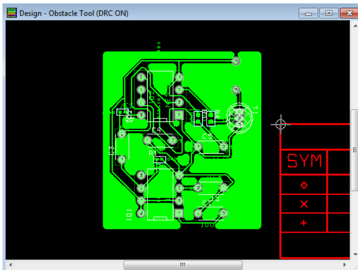
Obr. 4.19 Rozlévaná měď
