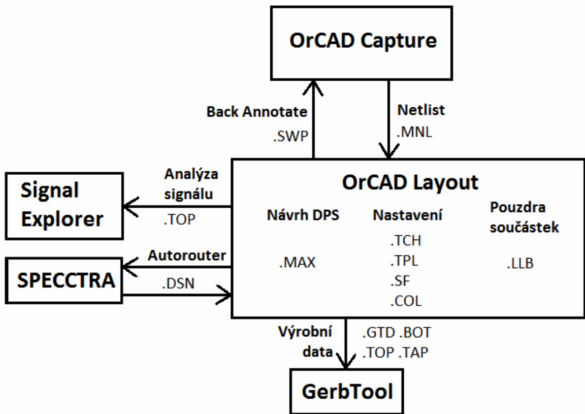
Obr. 3.2 Vazby jednotlivých souborů v OrCADu
