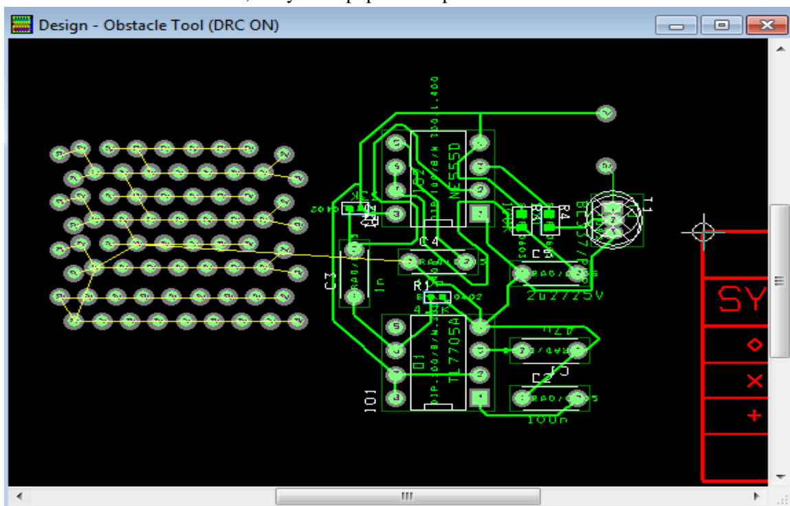
Obr. 4.20 Matice prokovů Free Via
