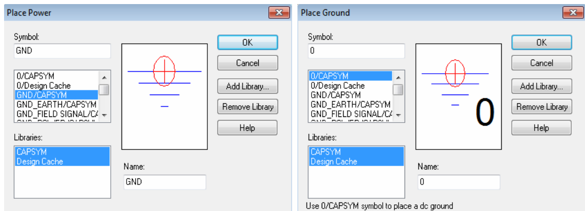
Obr. 4.4 Knihovny napájení
