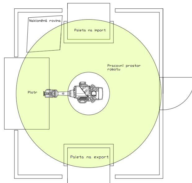
Obr. 6) Rozložení pracoviště
