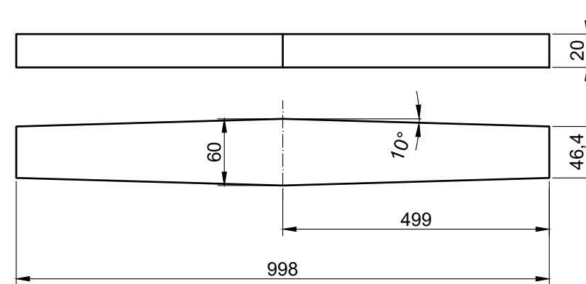
M 1:5
