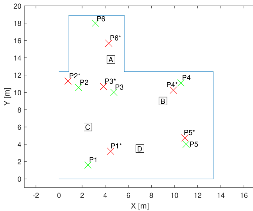
Obr. 6.9: Polohy lokalizovaných pozic v prostředí Aula – 4. varianta konfigurace (FLRC - BW = 300 kHz, BR = 260) (x – skutečná poloha, x – vypočtená poloha).
