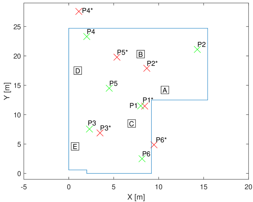
Obr. 6.26: Polohy lokalizovaných pozic v prostředí Šatna – 10. varianta konfigurace (LoRa ® - BW = 1600 kHz, SF = 12, P Tx = -18 dBm) (× – skutečná poloha, × – vypočtená poloha).
