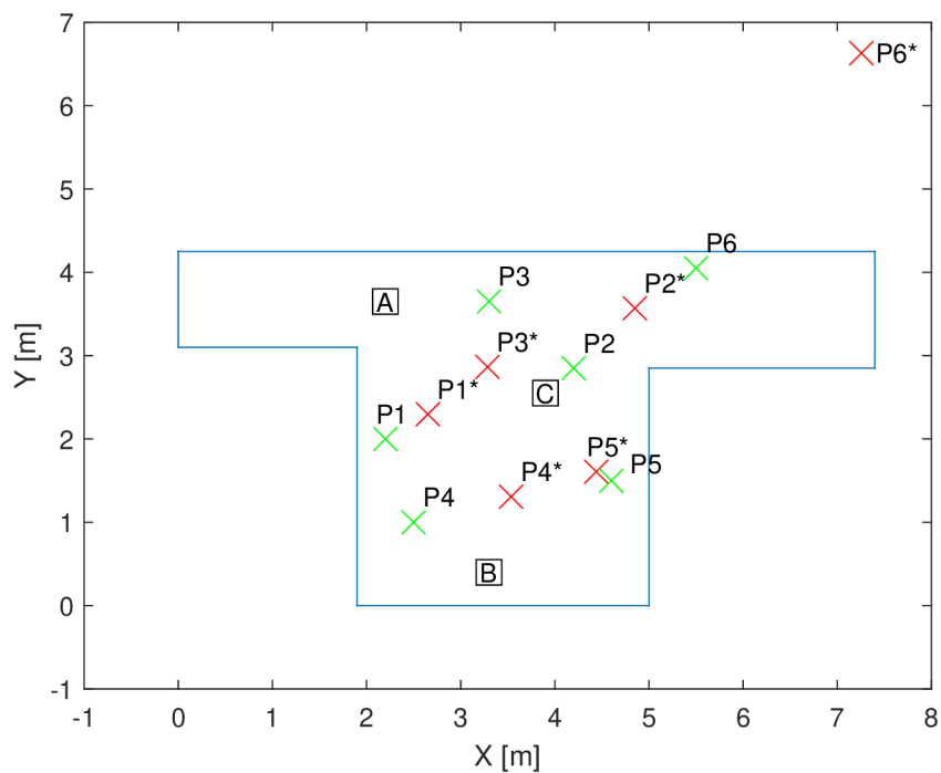
Obr. 5.5: Polohy lokalizovaných pozic v daném prostředí – 1. varianta konfigurace LoRa ® (BW = 800 kHz, SF = 12) (× – skutečná poloha, × – vypočtená poloha).
