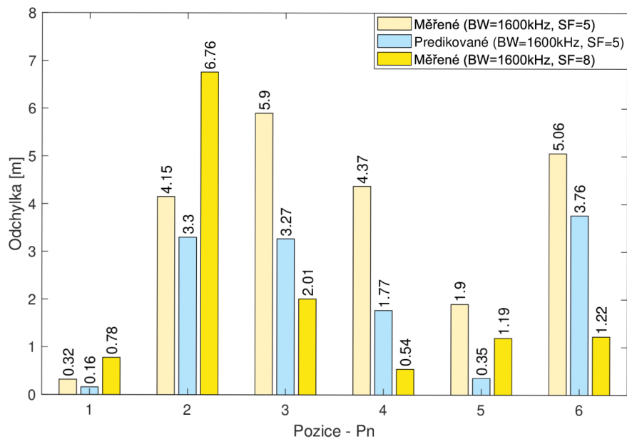
Obr. 6.40: Odchyly lokalizace v prostředí Šatna pro vybrané konfigurace.
