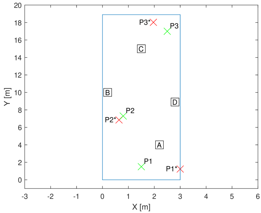
Obr. 6.33: Polohy lokalizovaných pozic v prostředí Chodba – 1. varianta konfigurace (LoRa ® - BW = 200 kHz, SF = 12) (x – skutečná poloha, x – vypočtená poloha).
