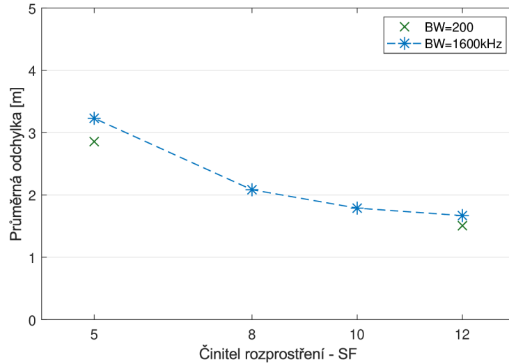
Obr. 6.28: Závislost průměrné odchylky lokalizace na hodnotě SF.
