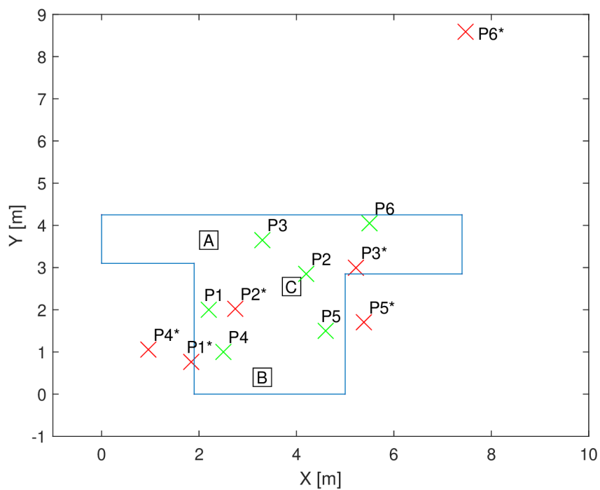
Obr. 5.6: Polohy lokalizovaných pozic v daném prostředí – 2. varianta konfigurace LoRa ® (BW = 1600 kHz, SF = 5) (× – skutečná poloha, × – vypočtená poloha).
