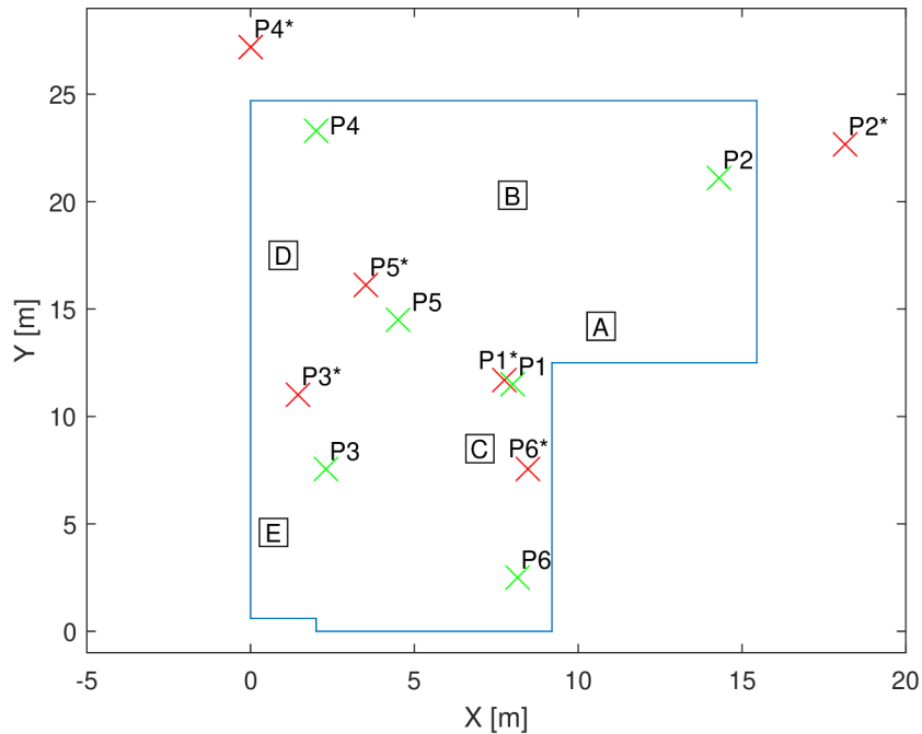
Obr. 6.20: Polohy lokalizovaných pozic v prostředí Šatna – 4. varianta konfigurace (LoRa ® - BW = 1600 kHz, SF = 5) (x – skutečná poloha, x – vypočtená poloha).
