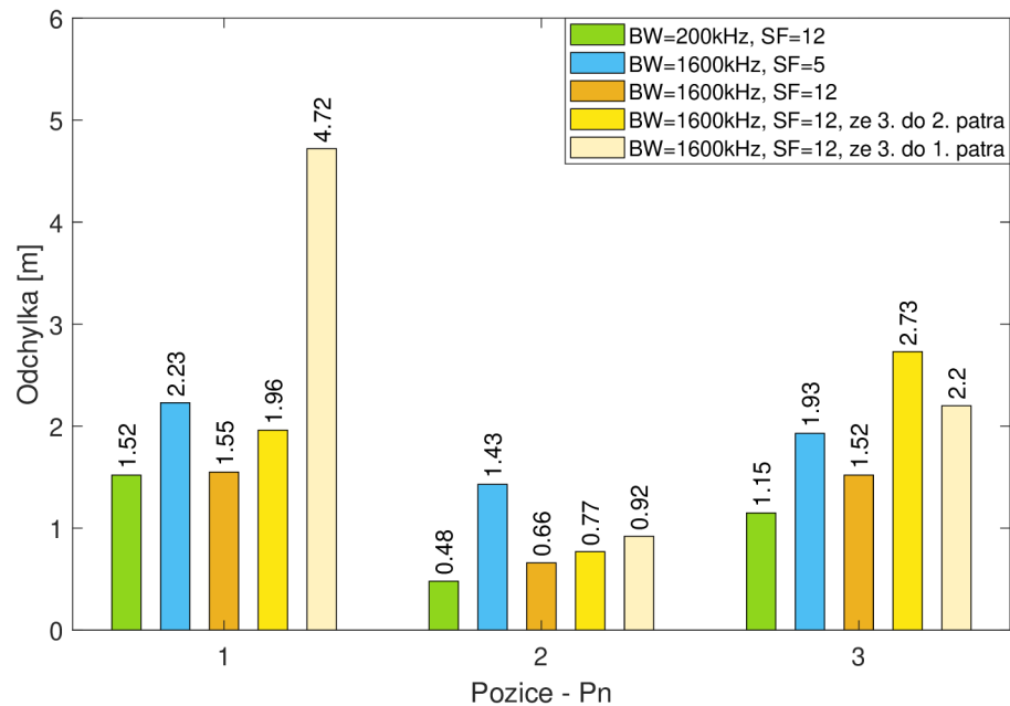
Obr. 6.38: Odchytky lokalizace jednotlivých pozic pro všechny varianty konfigurací v přenosovém prostředí – Chodba.
