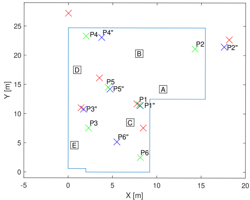
Obr. 6.39: Polohy lokalizovaných pozic v prostředí Šatna s využitím ML – konfigurace LoRa ® - BW = 1600 kHz, SF = 5 (x – skutečná poloha, x – původní vypočtená poloha, x – vypočtená poloha s využitím ML).
