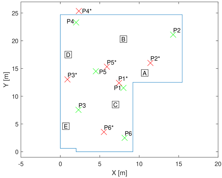
Obr. 6.25: Polohy lokalizovaných pozic v prostředí Šatna – 9. varianta konfigurace (LoRa ® - BW = 1600 kHz, SF = 12, P Tx = -8 dBm) (× – skutečná poloha, × – vypočtená poloha).
