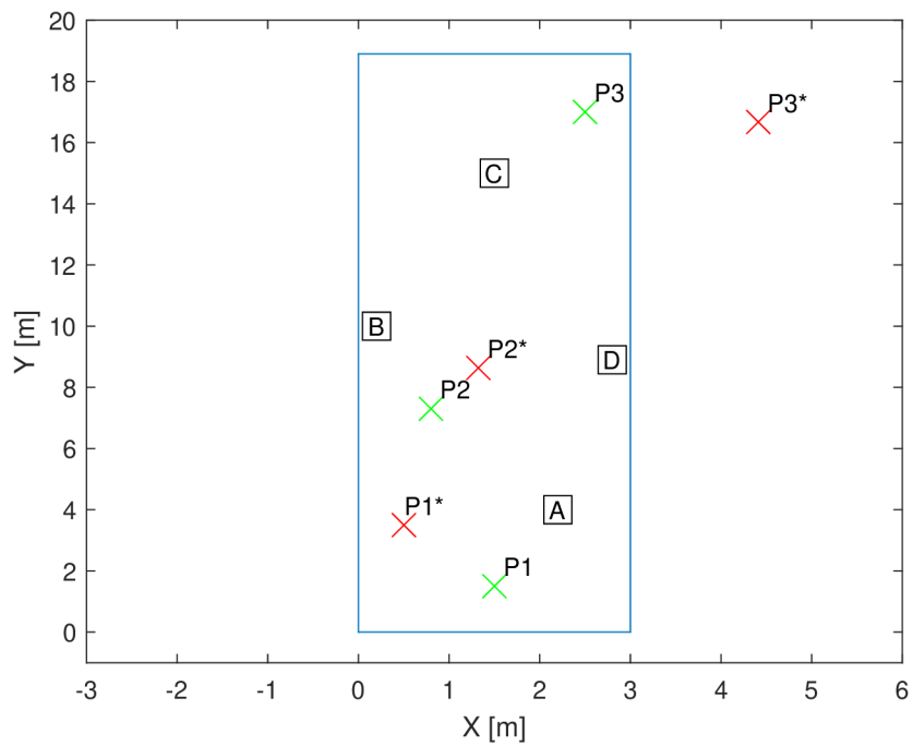
Obr. 6.34: Polohy lokalizovaných pozic v prostředí Chodba – 2. varianta konfigurace (LoRa ® - BW = 1600 kHz, SF = 5) (x – skutečná poloha, x – vypočtená poloha).
