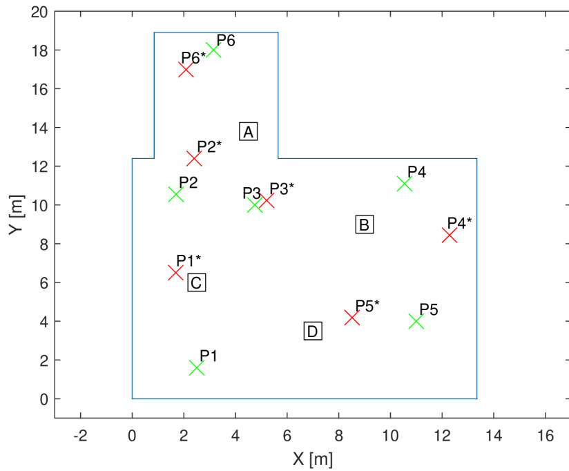
Obr. 6.8: Polohy lokalizovaných pozic v prostředí Aula – 3. varianta konfigurace (FLRC - BW = 1200 kHz, BR = 1300) (x – skutečná poloha, x – vypočtená poloha).
