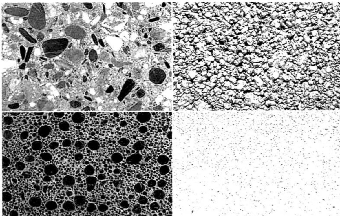
Obr. 2 Pohled na řezy různými lehkými betony
