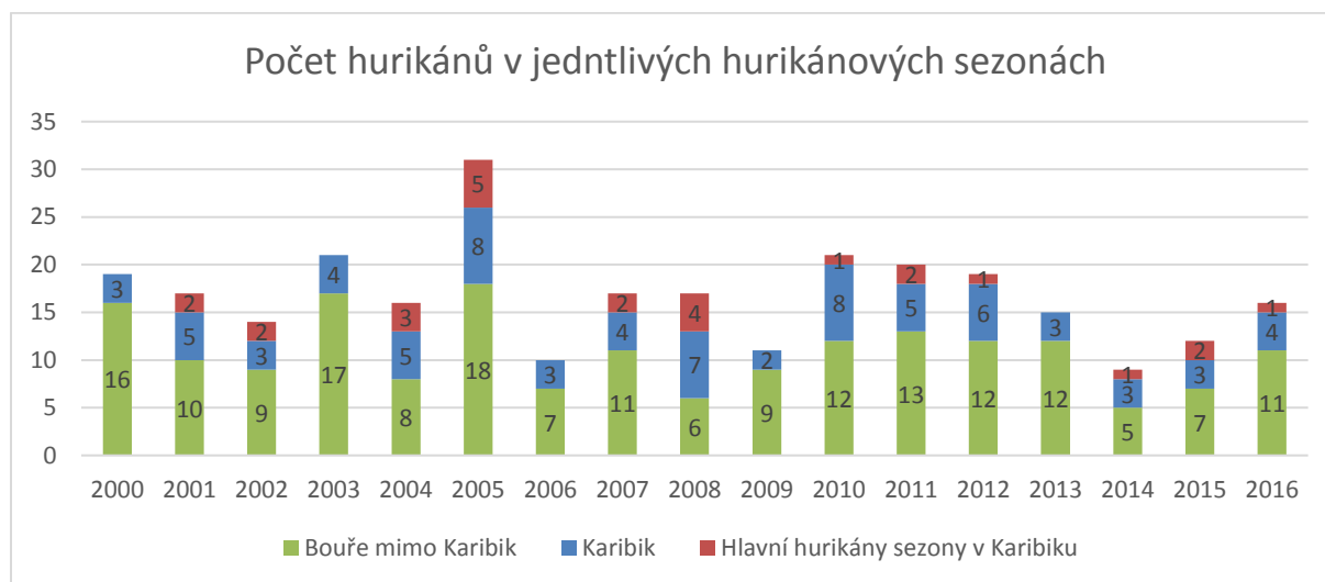
Graf. č. 4: Intenzita hurikánových sezon v letech
