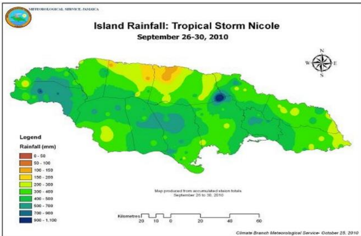
Příloha č. 4: Prostorová analýza srážkových úhrnů na Jamajce při přechodu tropické bouře Nicole v roce 2010
