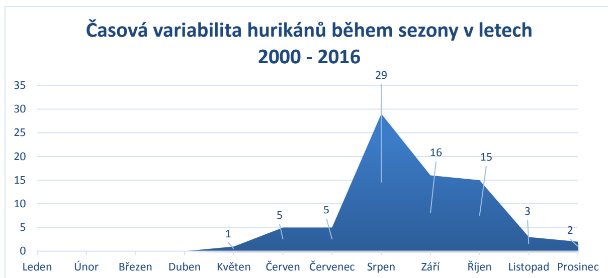
Graf č. 5: Časová variabilita hurikánů během sezony, období 2000 - 2016
