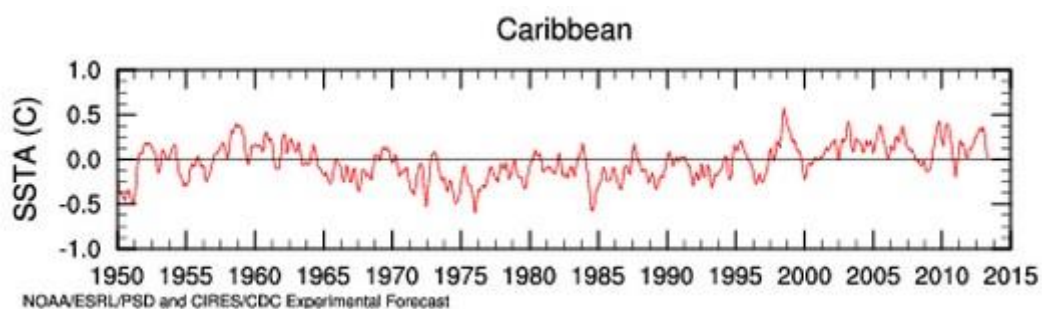
Graf č. 3: Odchylka teploty moří v Karibském moři, 1950 - 2015
