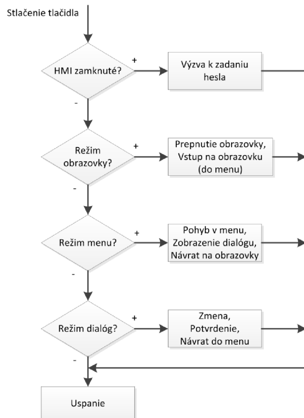
Obr. 9.1: Vývojový diagram grafickej časti
