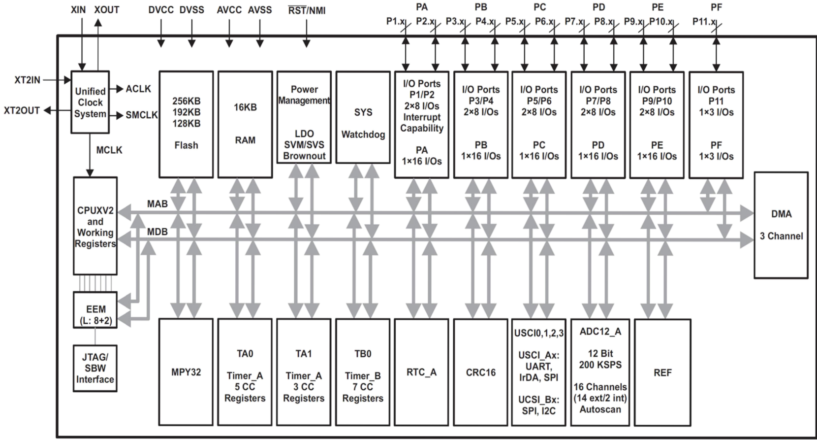
Obr. 4.1: Bloková schéma MSP430F5438A [5]
