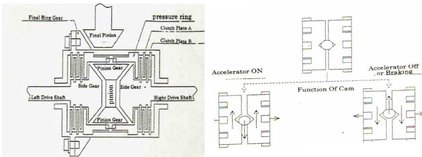
Obr. 11 Schéma LSD diferenciálu[9]
