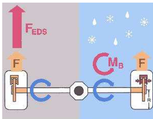
Obr. 22 Vyvolaný brzdny moment
