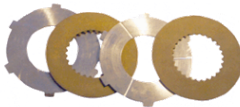
Obr. 20 Lamely diferenciálu [7]
