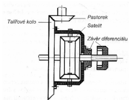
Obr. 5 Schématický závěr diferenciálu[3]
