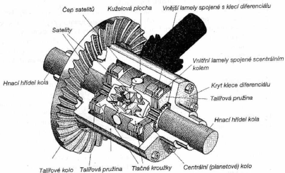
Obr. 15 Samosvorný diferenciál s třecí lamelovou spojkou [3]
