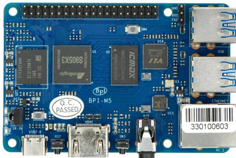
Obrázek 7: Počítač Banana Pi M5 [20]
